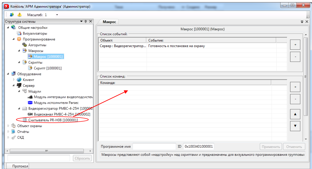
Рис. 80 Добавление команды в макрос с помощью перетаскивания объекта мышью
