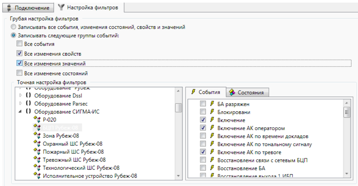
Рис. 123. Окно точной настройки фильтров
