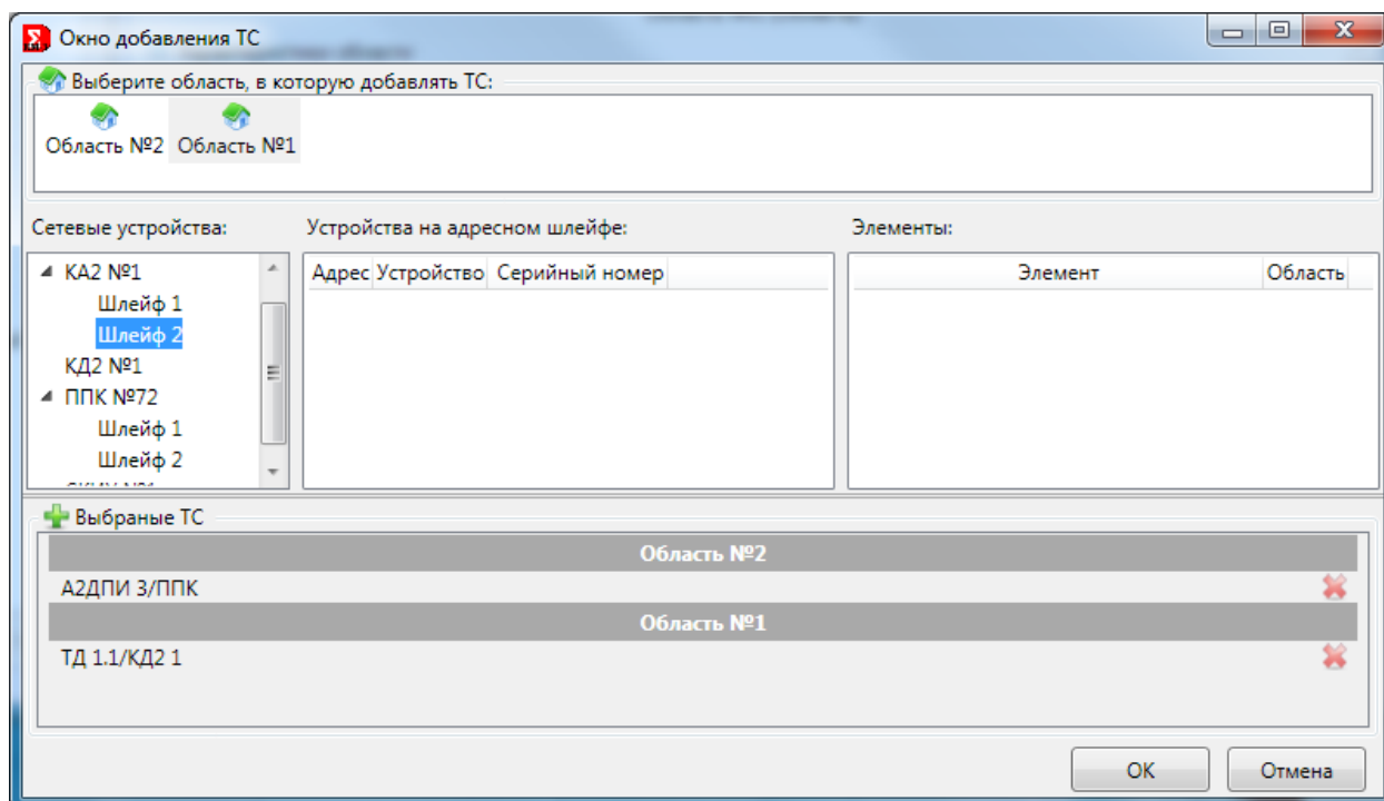
Рис. 285 Выбор ТС для добавления
