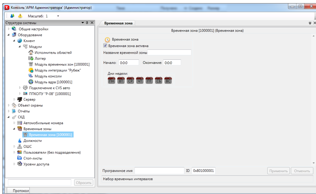
Рис. 64 Редактор временных зон
