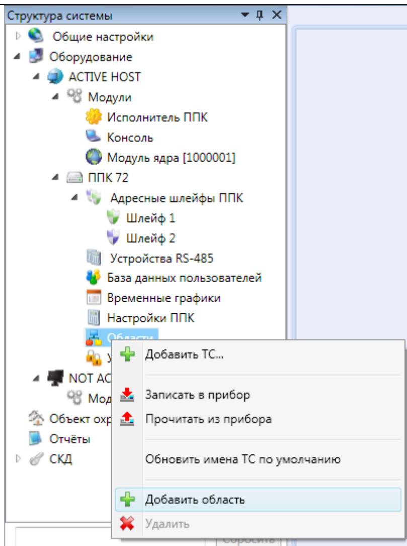
Рис. 271 Добавление области ППК
