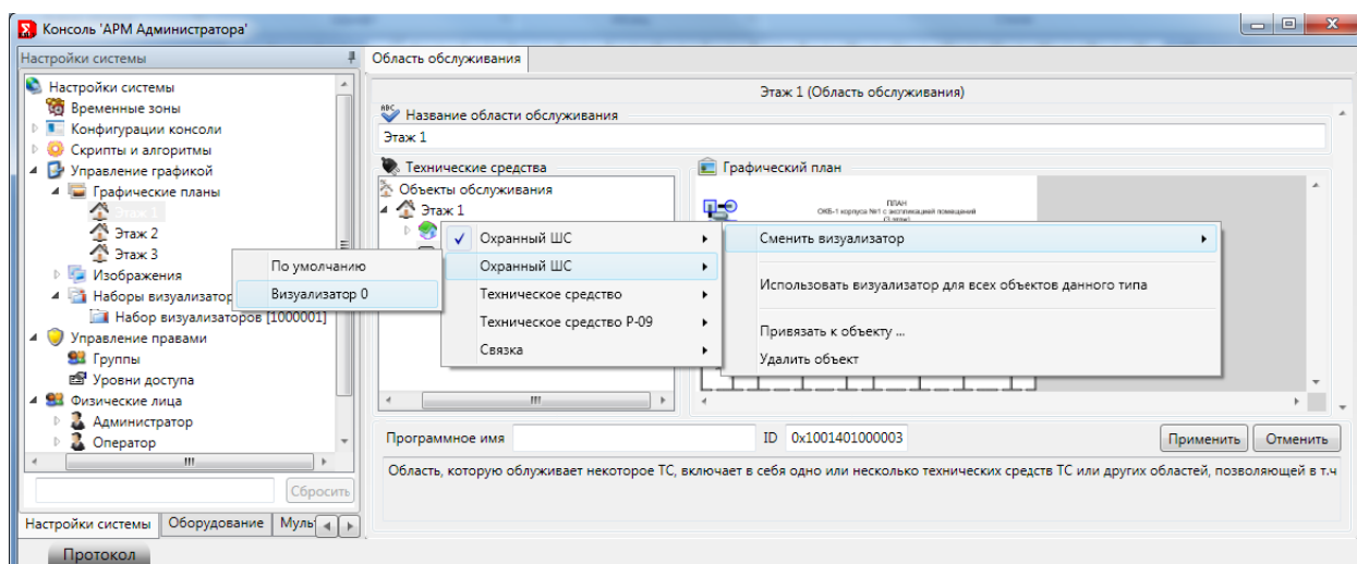
Рис. 112 Смена визуализатора объекта на ГП. Выбор визуализатора
