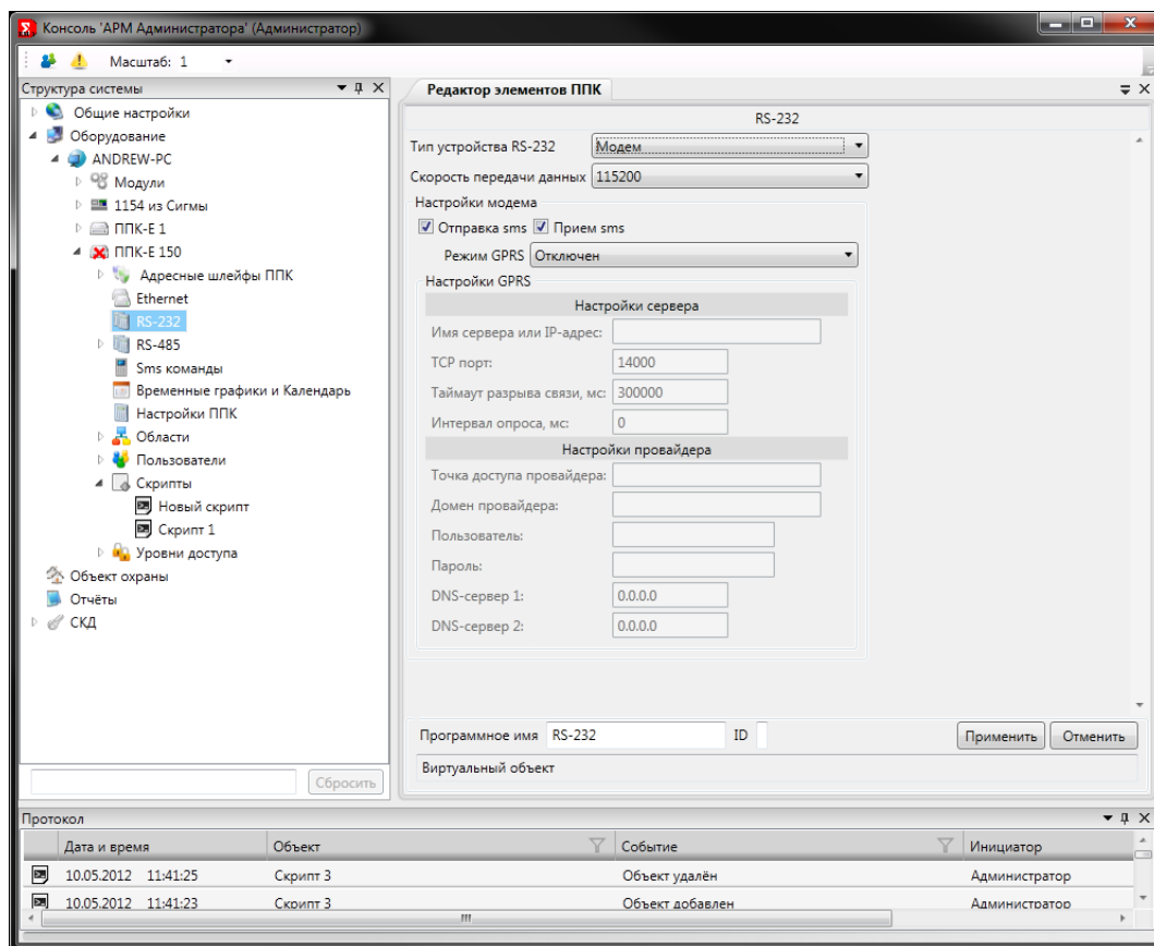
Рис. 300 Редактирование настроек RS-232 ППК
