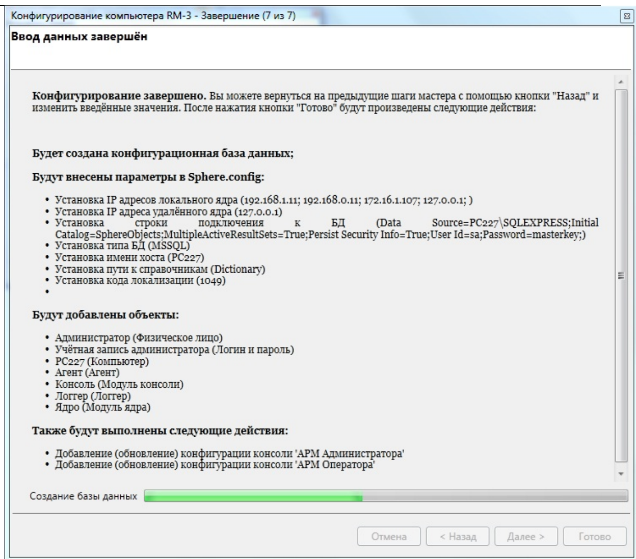
Рис. 27 Мастер конфигурирования RM-3. Процесс создания конфигурации компьютера.
