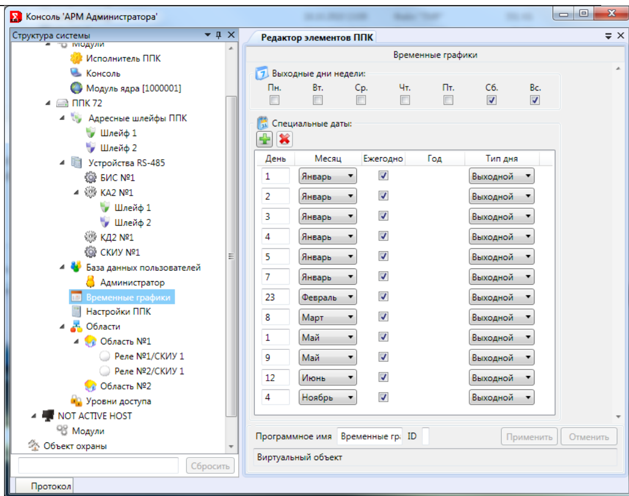
Рис. 289 Редактирование календаря RM-3
