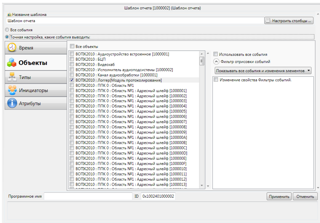
Рис. 128. Вкладка выбора событий для отчёта
