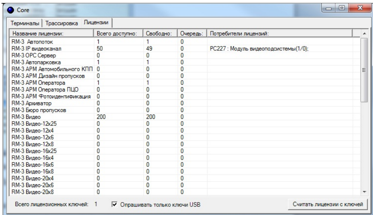
Рис. 41. Окно ядра. Лицензии.
