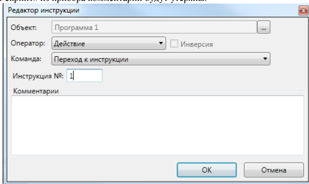
Рис. 221 Редактор инструкций
