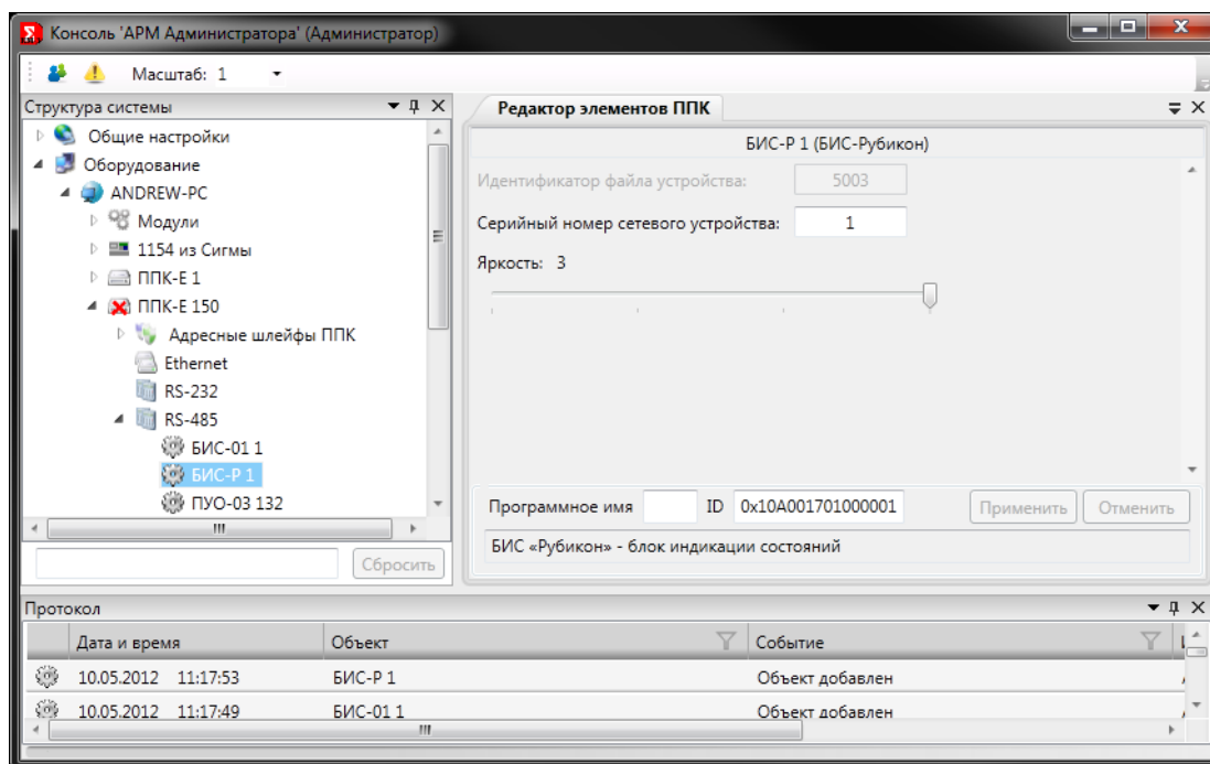
Рис. 276 Настройки БИС-Рубикон
