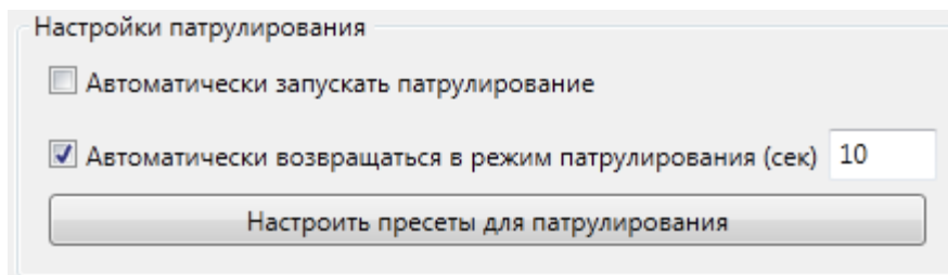
Рисунок 184– Настройки патрулирования.
