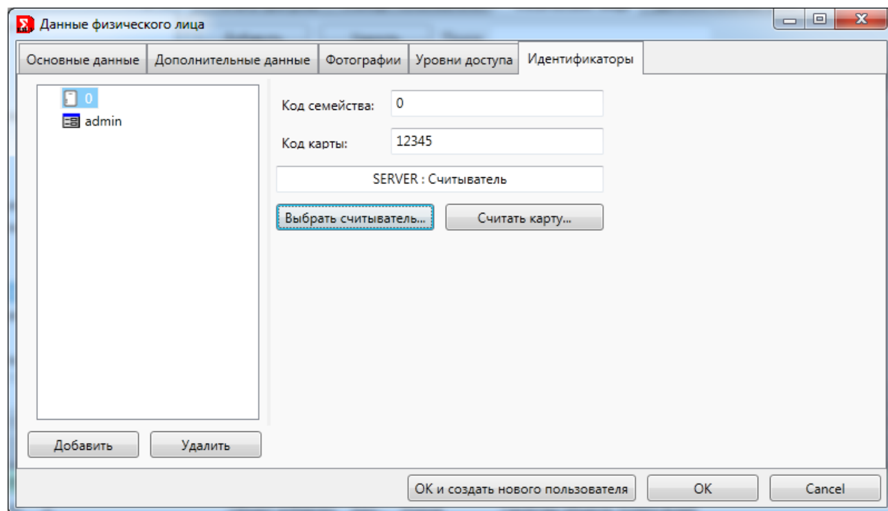
Рис. 319 – Считывание карты
