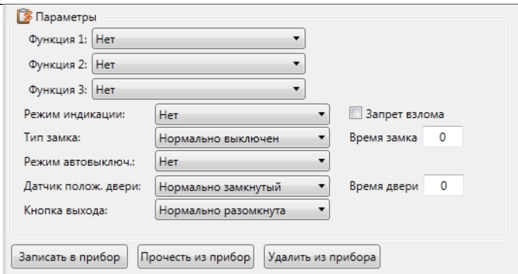
Рис. 251 Параметры УСК-02С
