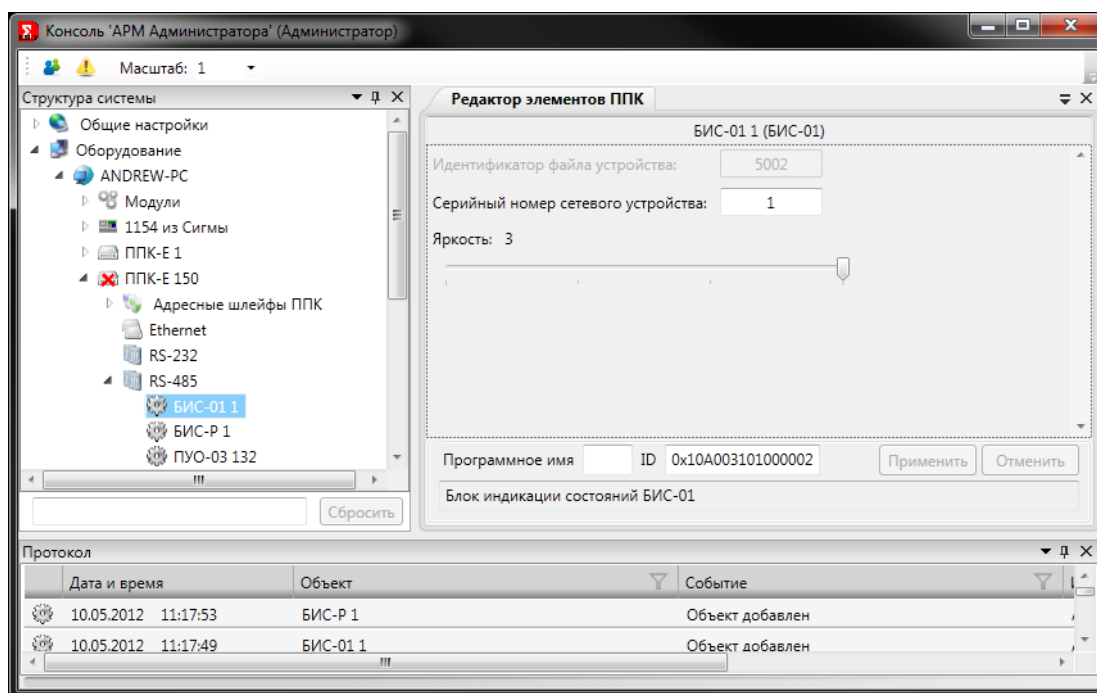
Рис. 277 Настройки БИС-01
