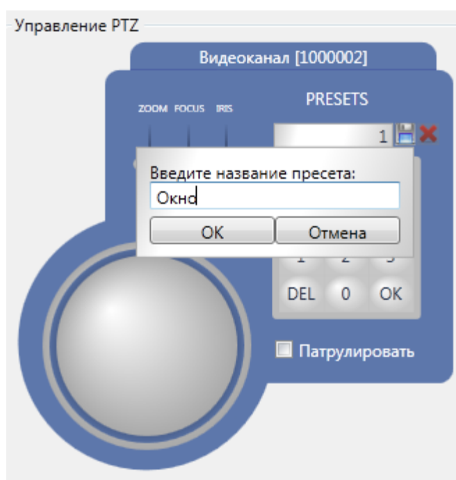
Рисунок 182– Создание пресета
