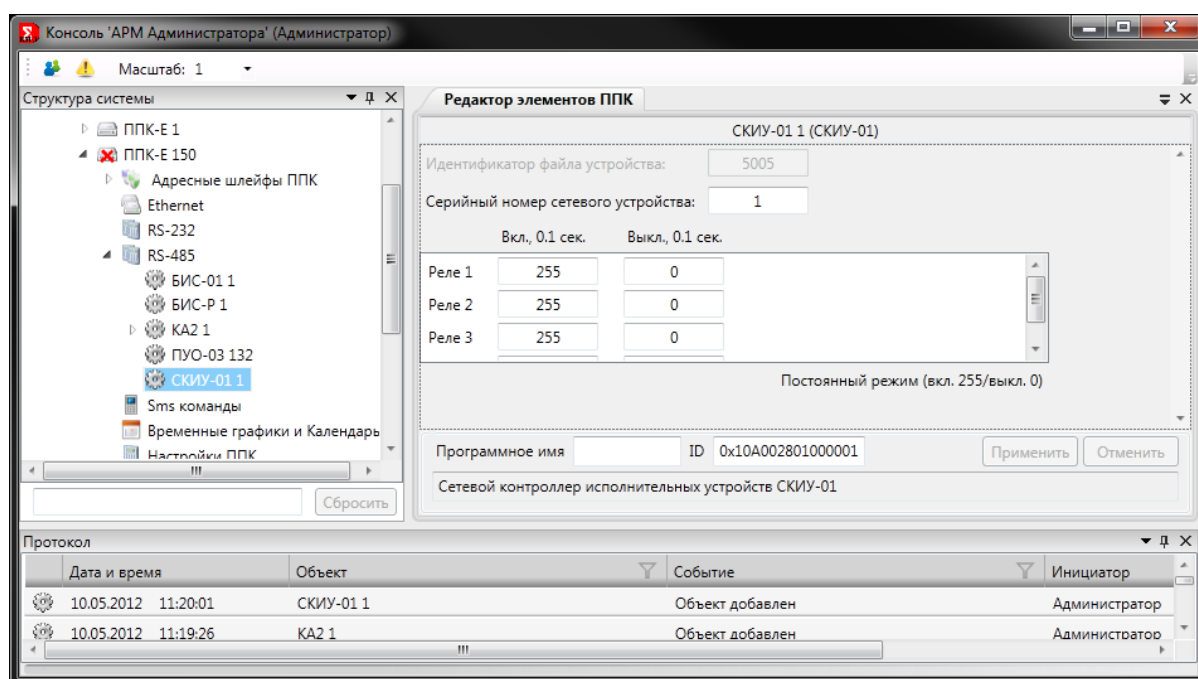
Рис. 280 Настройки СКИУ-01
