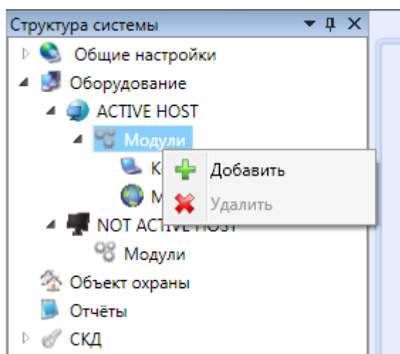
Рис. 254 Добавление модуля
