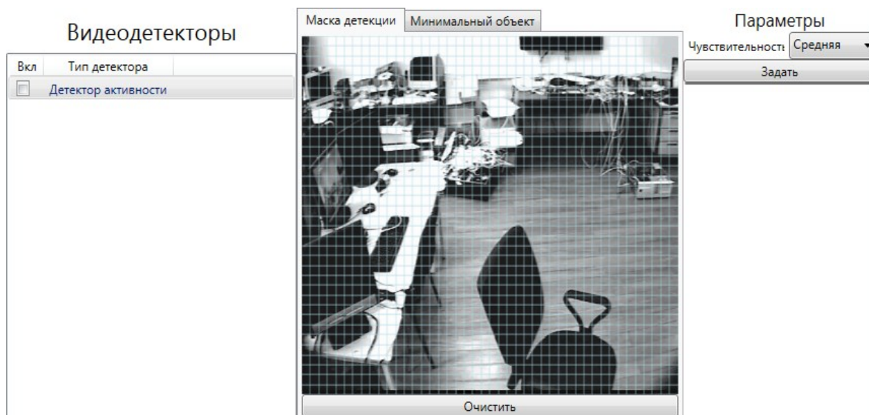
Рис. 152 Настройка видеодетекторов.
