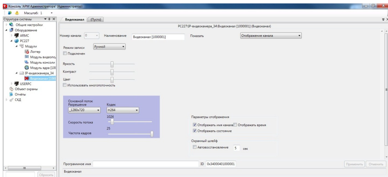
Рис. 144 Настройки видеоканала.
