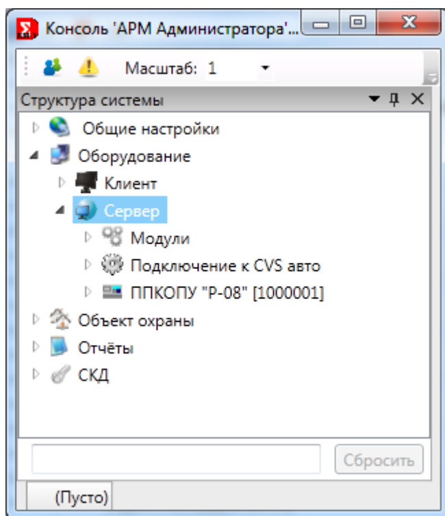
Рис. 137 Дерево оборудования
