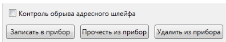
Рис. 240 Параметры СКАШ
