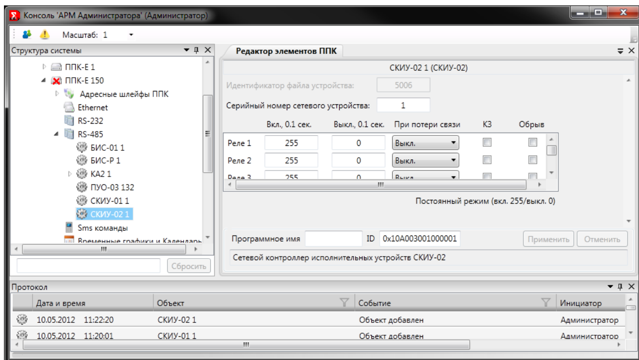
Рис. 281 Настройки СКИУ-02
