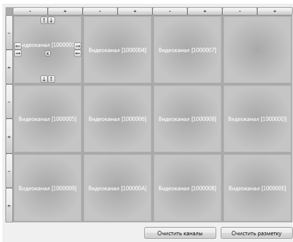
Рис. 163 Конструктор видеообласти.
