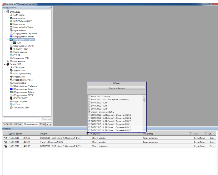
Рис 136 Использование фильтров
