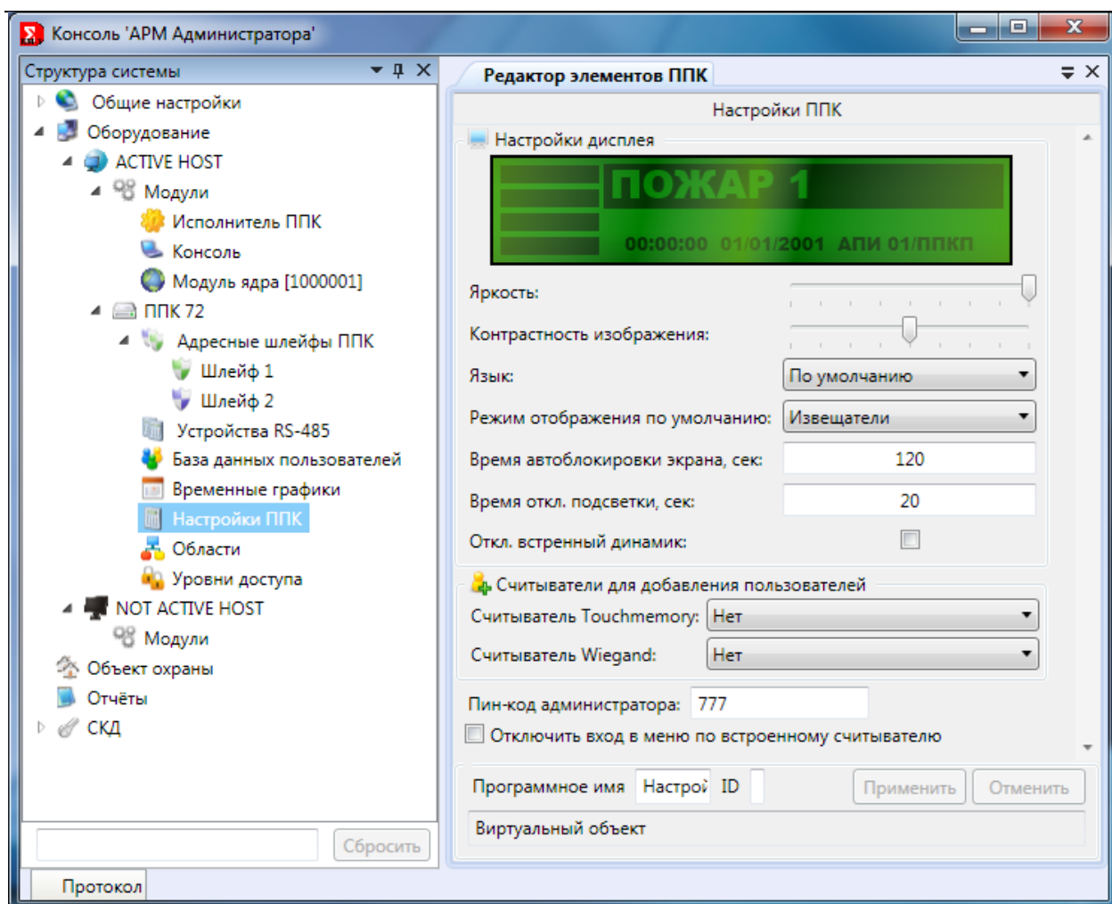
Рис. 270 Настройка ППК
