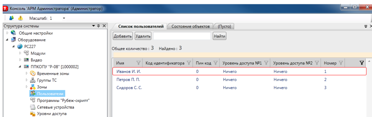
Рис. 217 Список пользователей
