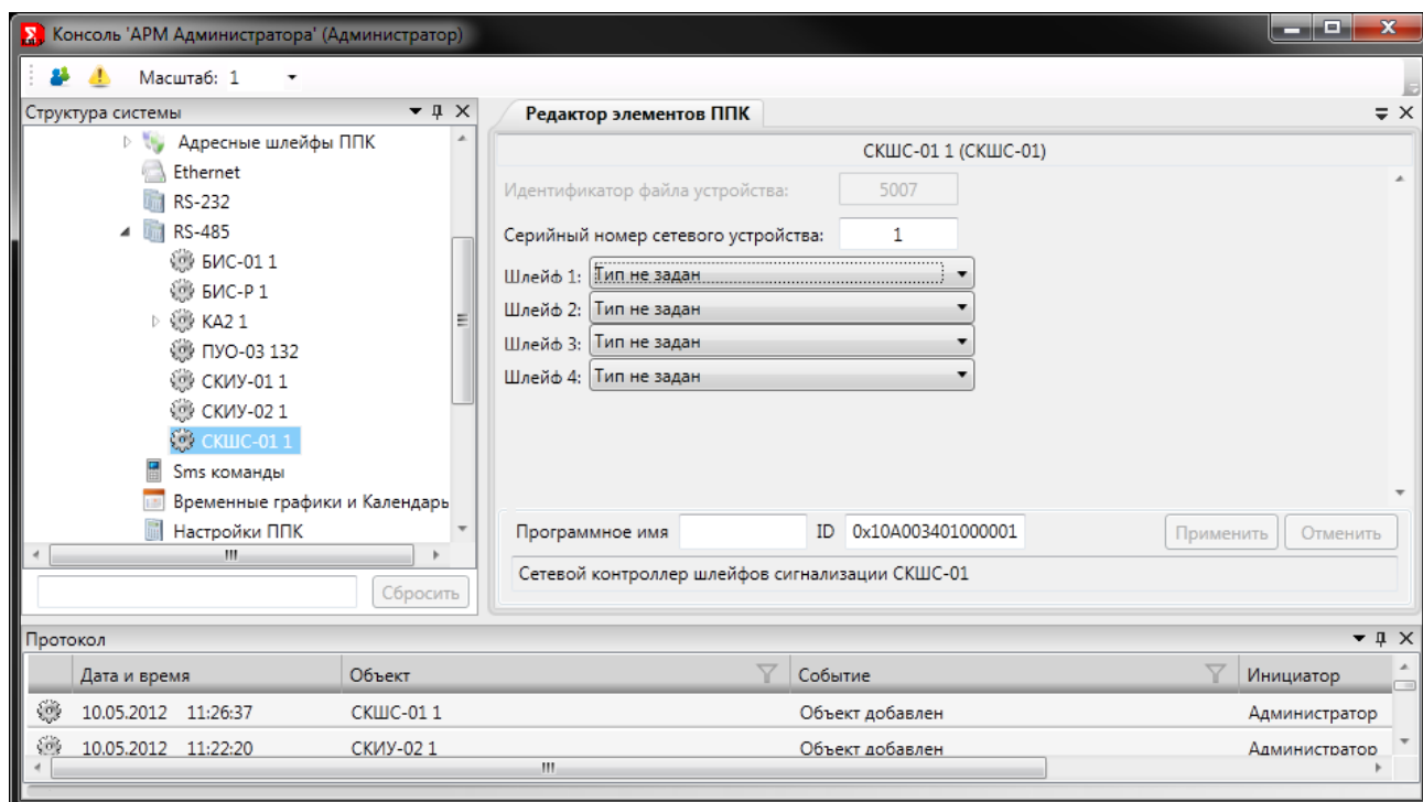
Рис. 282 Настройки СКШС-01
