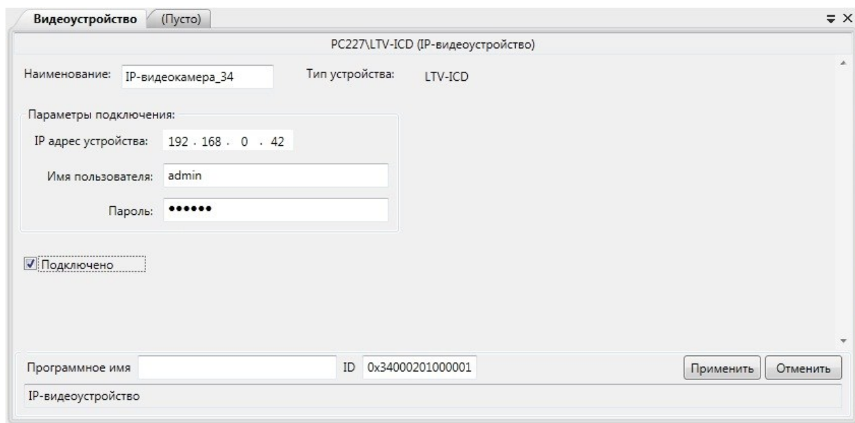
Рис. 143 Настройки видеоустройства.
