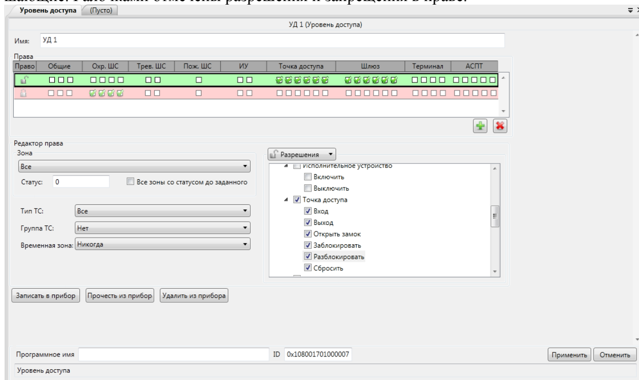
Рис. 253 Редактор уровня доступа
