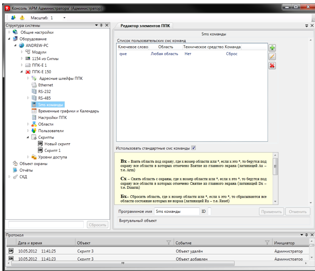
Рис. 301 Редактирование настроек sms команд ППК
