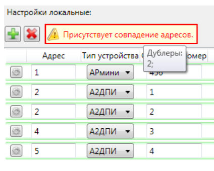
Рис. 268 Подробности о дублированных адресах
