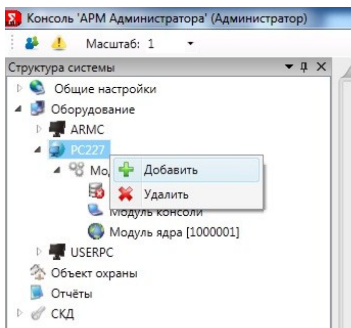
Рис. 138 Конфигурировании системы
