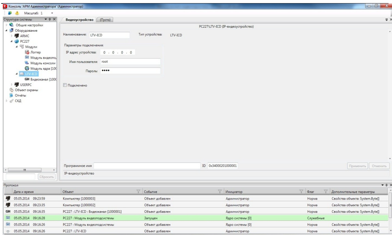
Рис. 142 Подключение видеоустройства.
