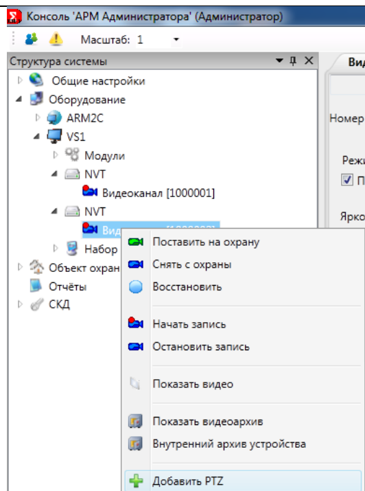
Рисунок 179– Добавление PTZ
