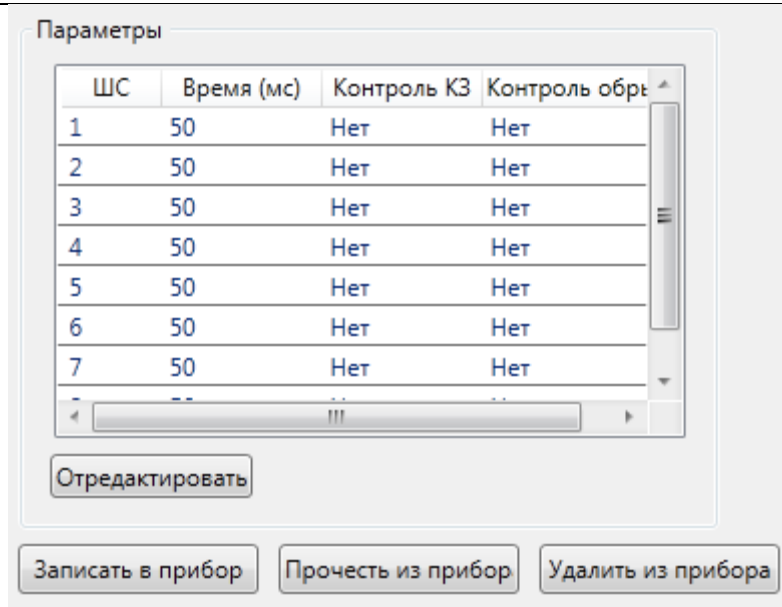
Рис. 247 Параметры СКШС-03
