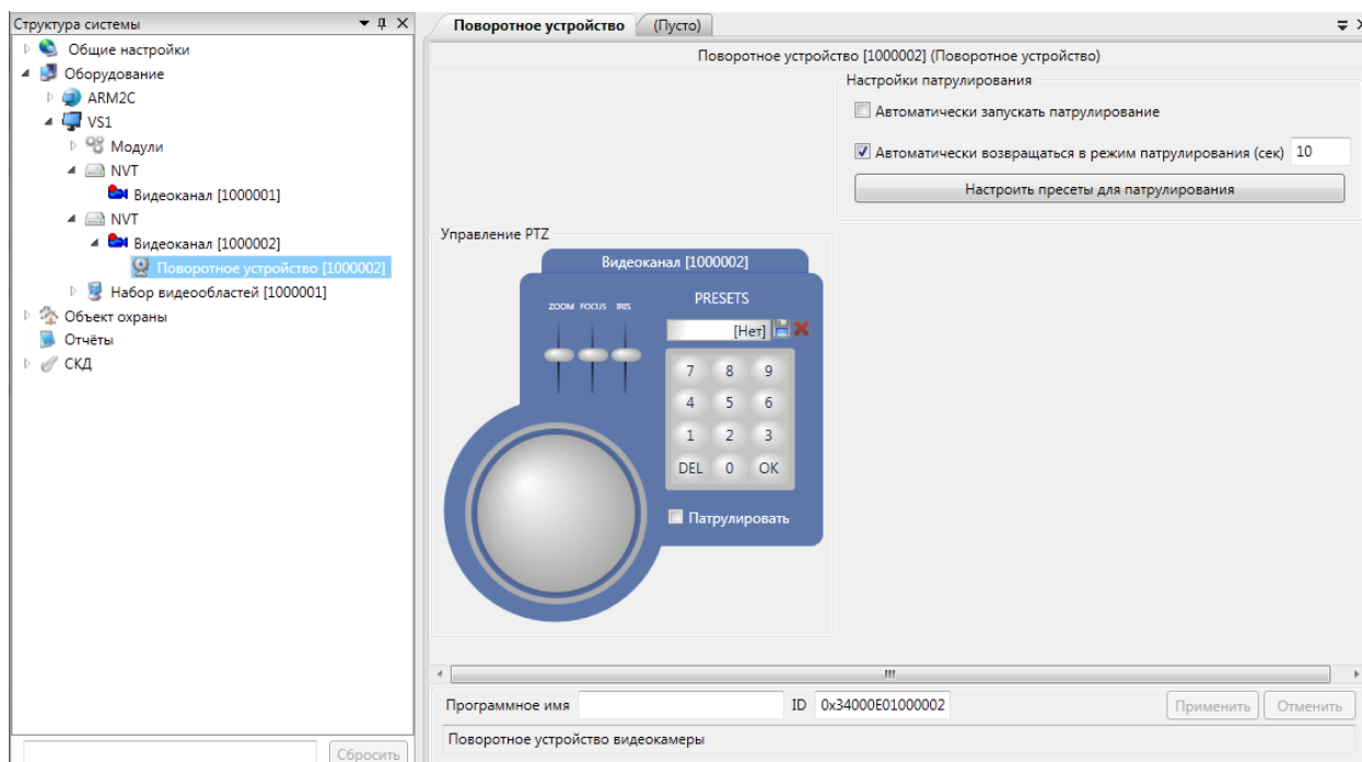
Рисунок 180 – Конфигурирование PTZ
