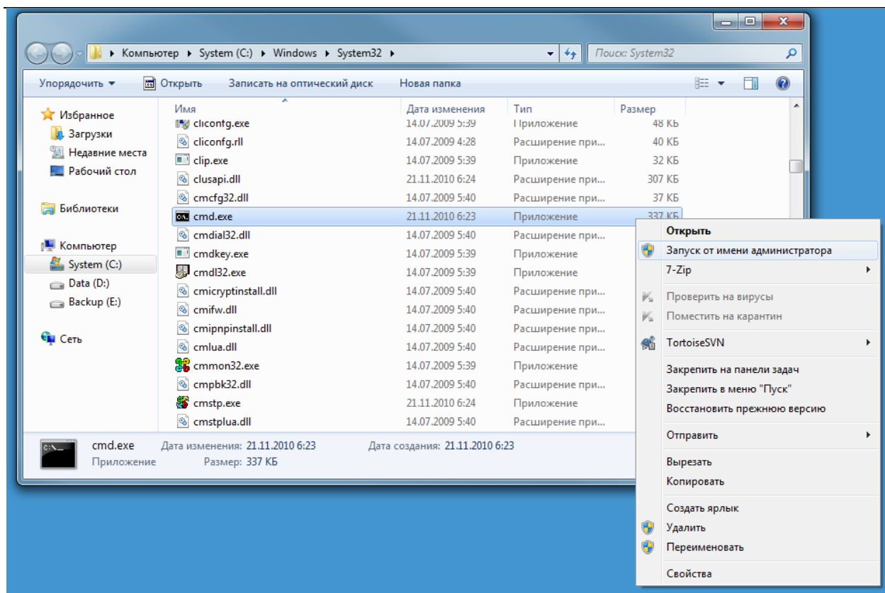
Рис. 304 – Запуск cmd.exe.
