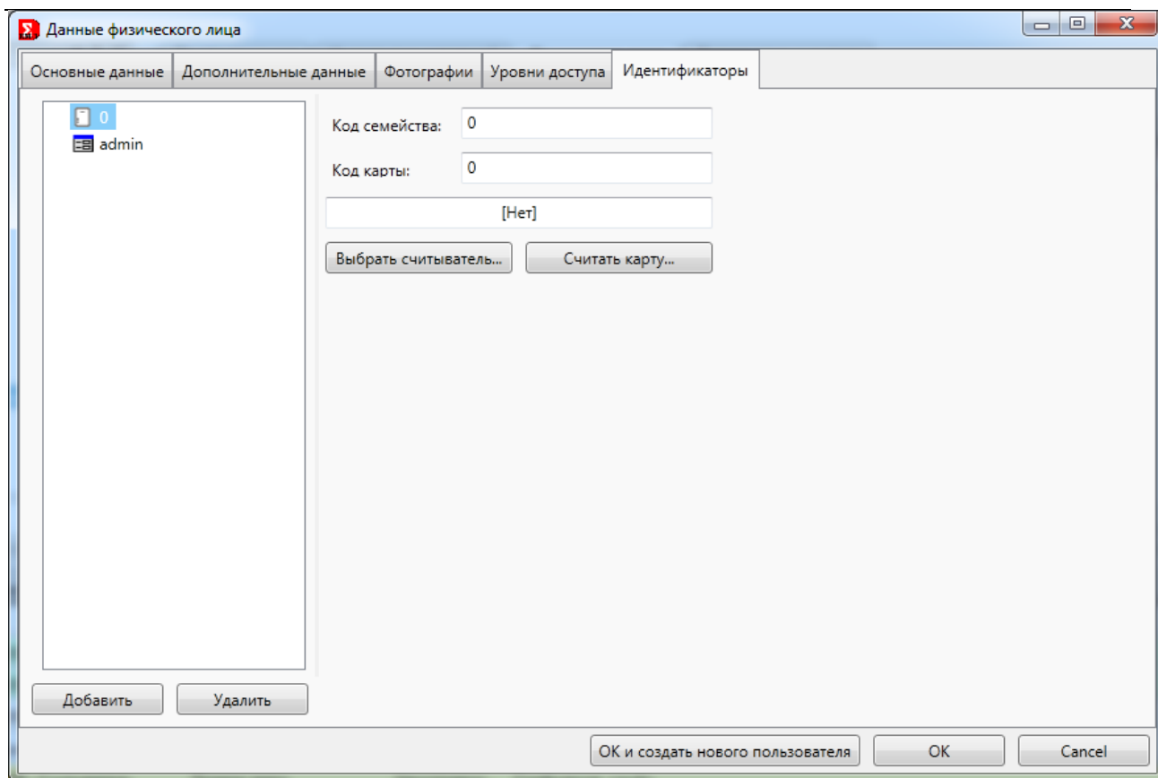
Рис. 317 – Редактор карты
