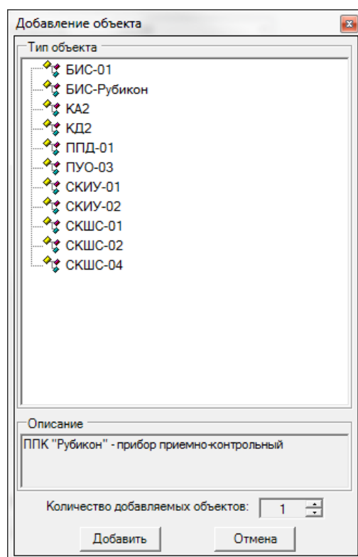
Рис. 275 Устройства RS-485
