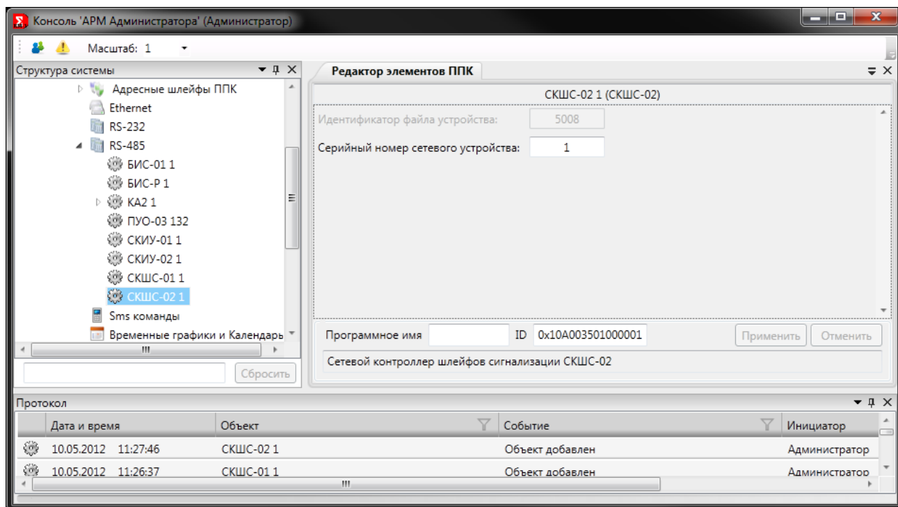
Рис. 283 Настройки СКШС-02
