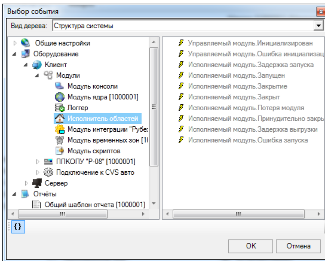
Рис. 69 Выбор события
