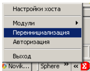
Рис. 119. Переинициализация Агента
