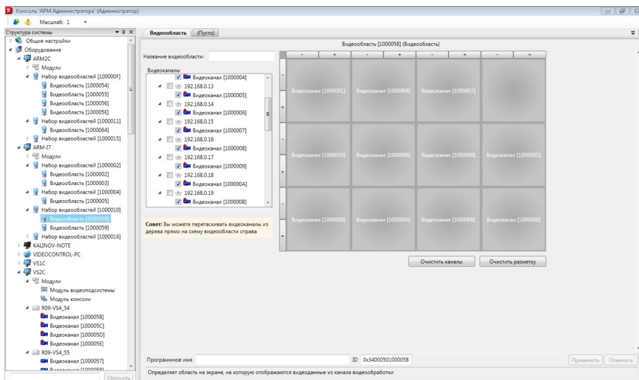
Рис. 162 Редактор видеообласти.
