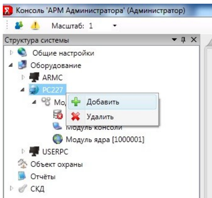
Рис. 158 Конфигурировании системы.
