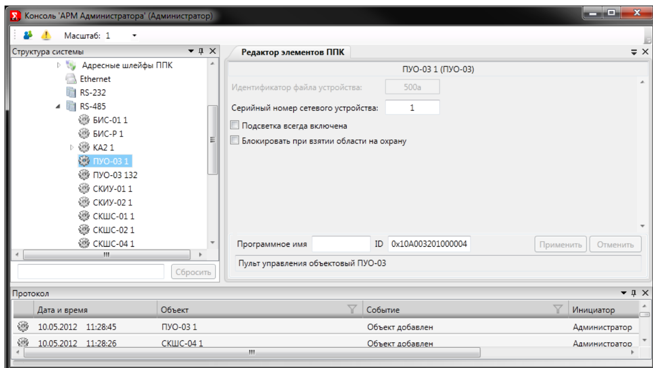
Рис. 284 Настройки ПУО-03
