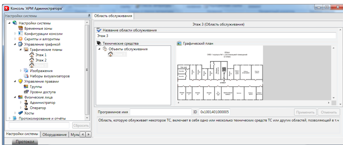
Рис. 90 Графический план
