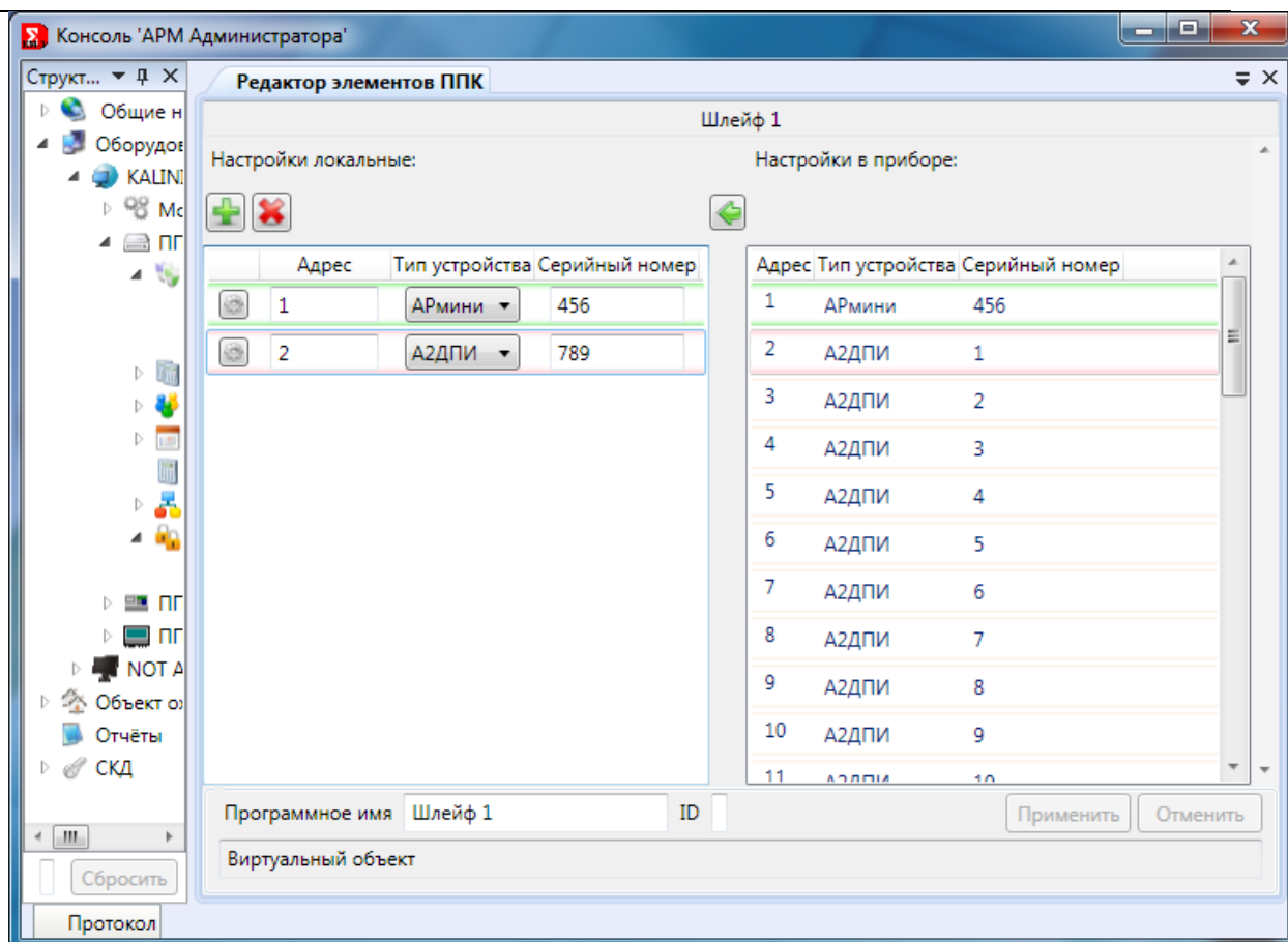
Рис. 266 Сравнение устройств на ПК и в приборе
