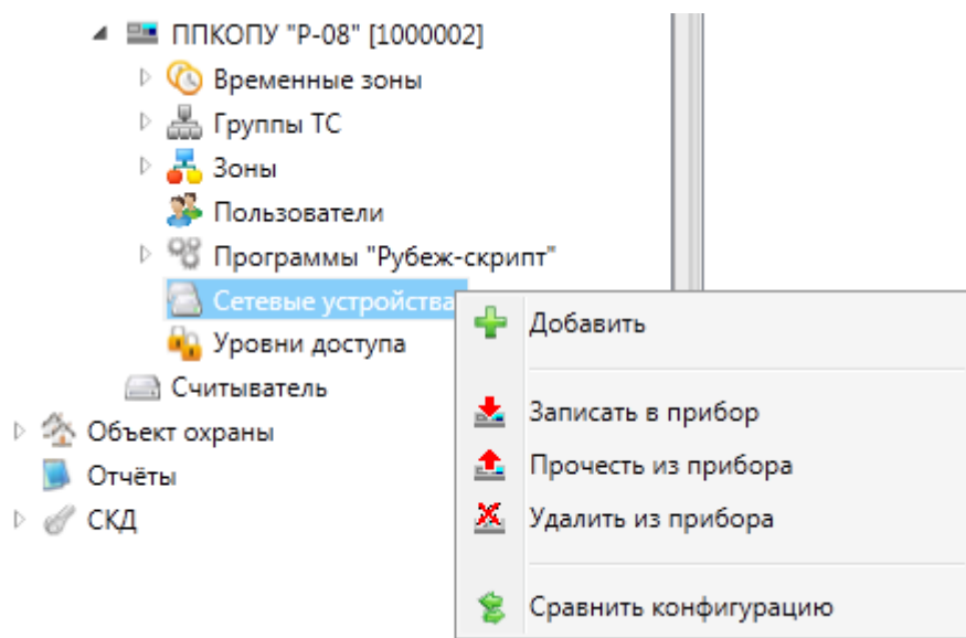
Рис. 224 Контекстное меню списка СУ
