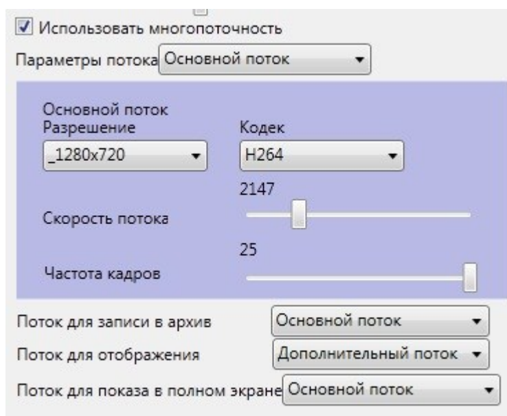
Рис. 148 Настройки видеоканала. Многопоточность.
