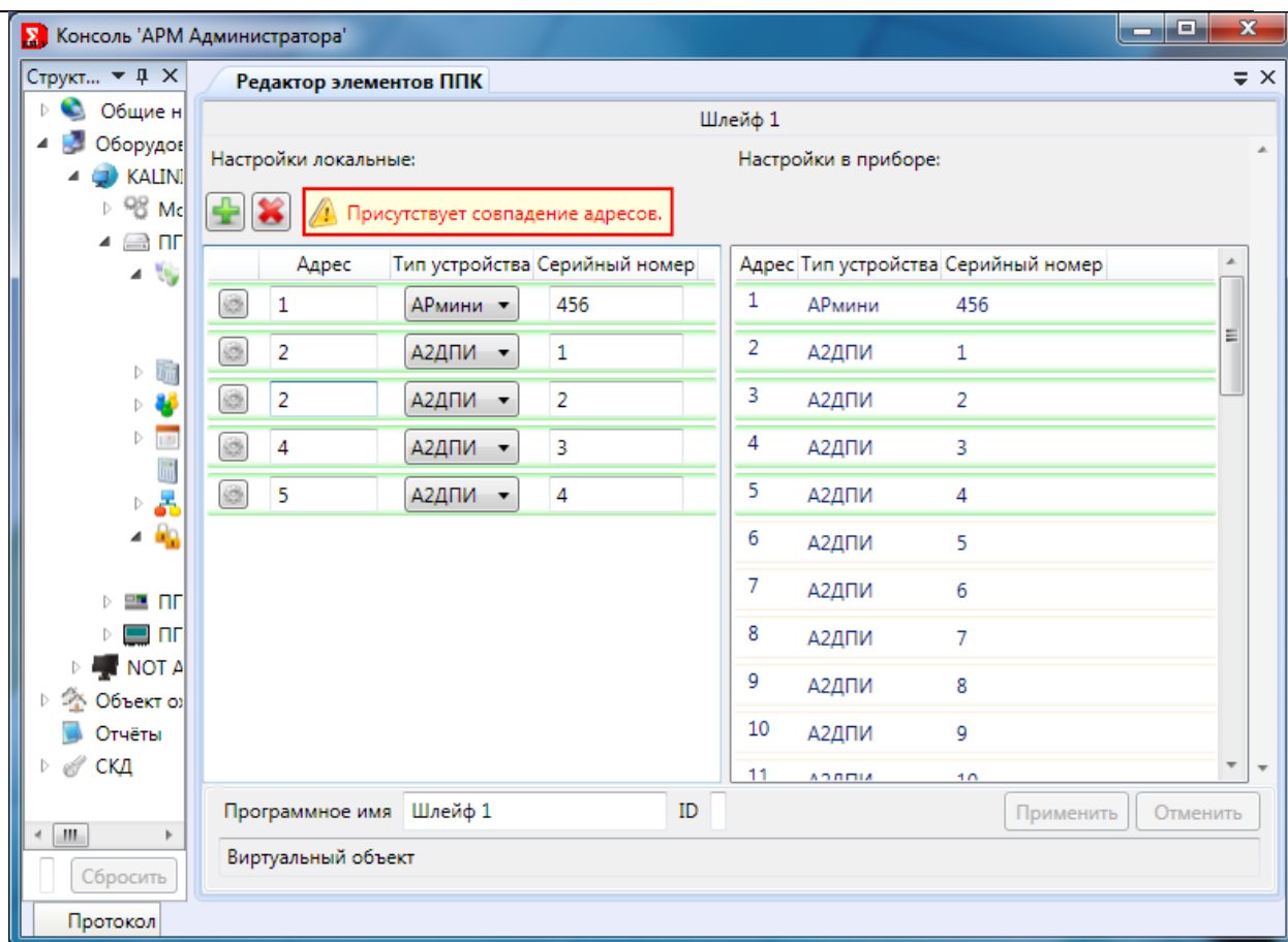
Рис. 267 Совпадение адресов адресных устройств
