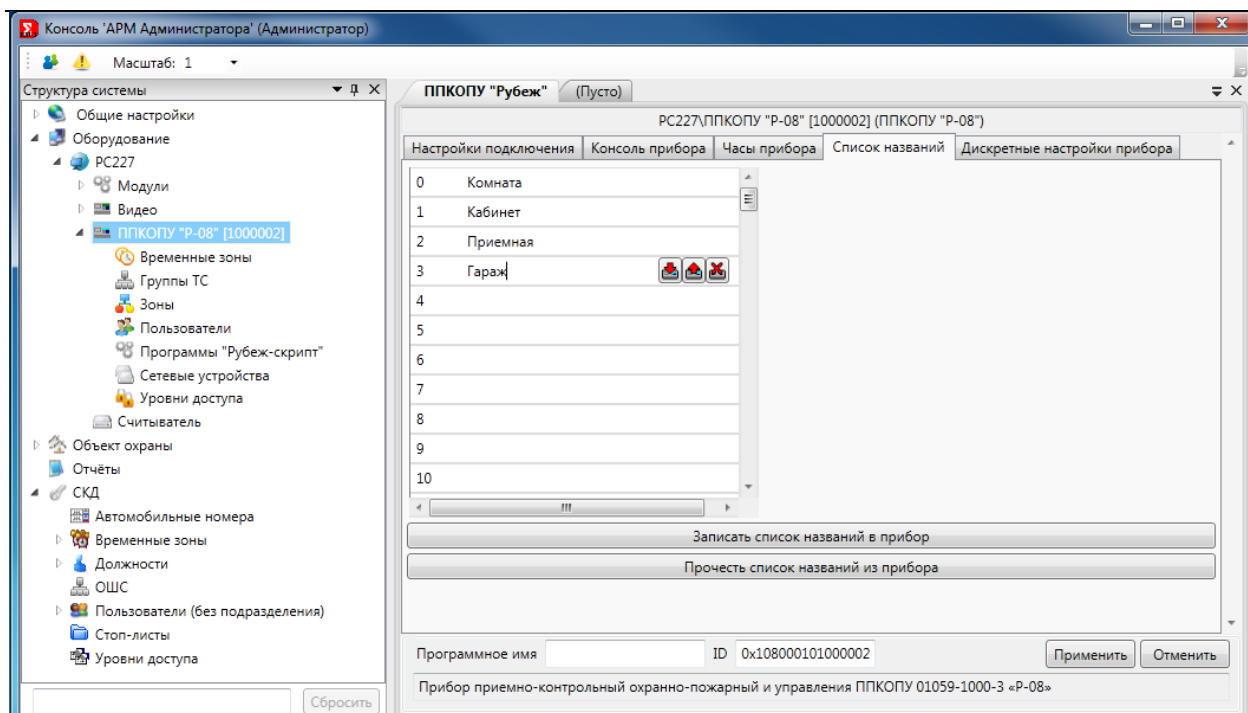
Рис. 194 Вкладка «Список названий»
