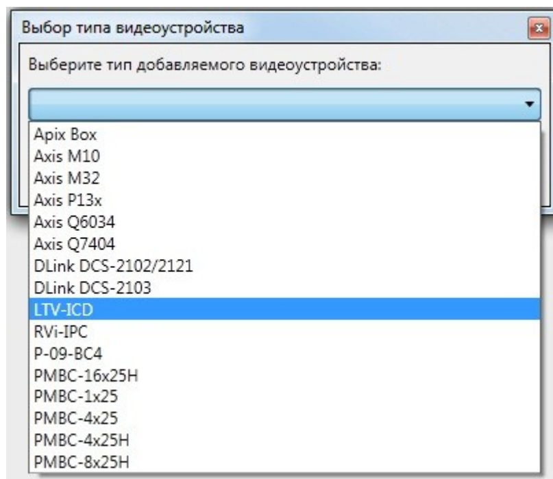
Рис. 141 Список поддерживаемых видеоустройств.
