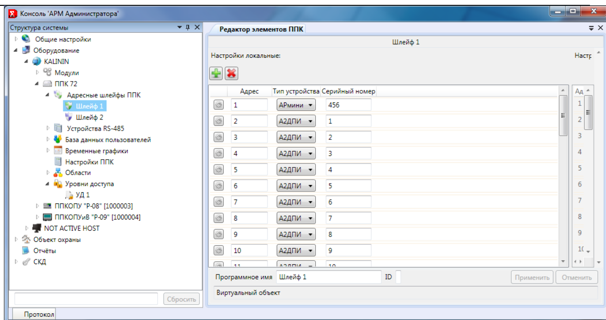
Рис. 265 Настройка устройств на адресных шлейфах RM-3
