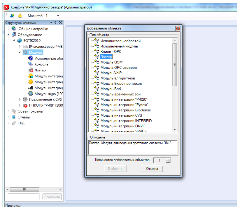
Рис. 117. Добавление модуля Логгера
