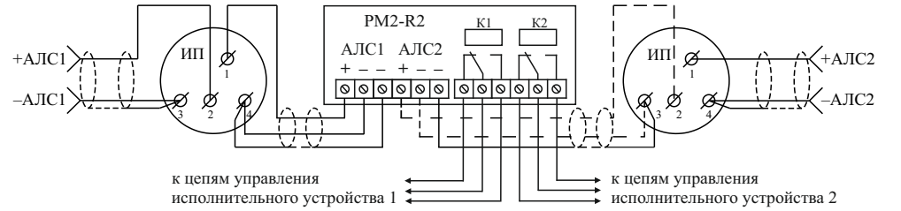
Рисунок 6 – Подключение релейного модуля PM2-R2 к АЛС кольцевого типа
