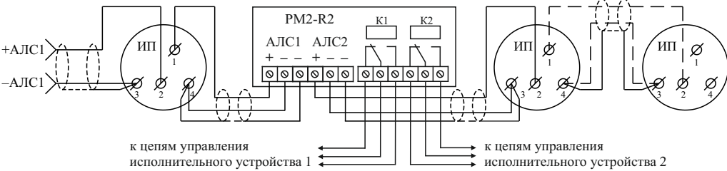
Рисунок 5 – Подключение релейного модуля PM2-R2 к АЛС радиального типа
