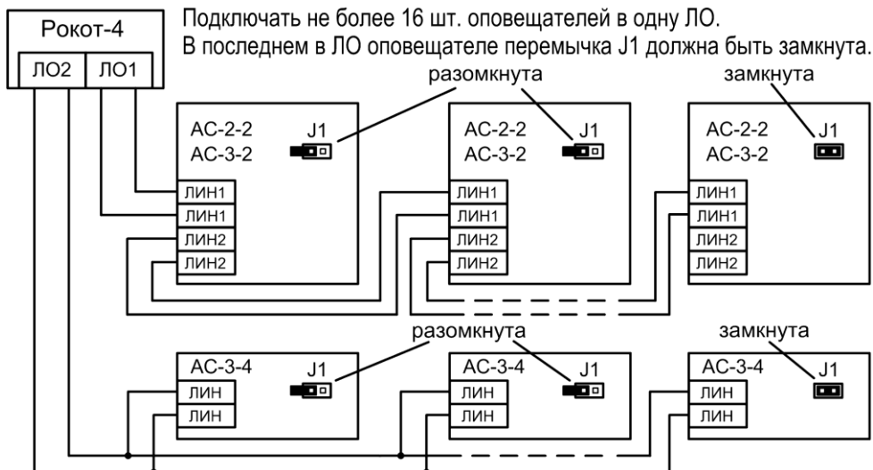
Рис.А4 Схема подключения оповещателей «AC-2-2», «AC-3-2» и «AC-3-4» (параллельное соединение)
