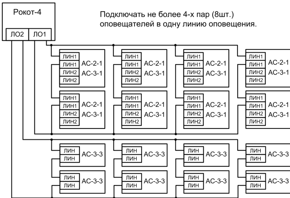
Рис.А3 Схема подключения оповещателей «AC-2-1», «AC-3-1» и «AC-3-3» (параллельно-последовательное соединение)
