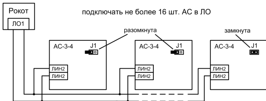
Рис.А6 Схема подключения акустических систем «АС-3-4» (параллельное соединение)
