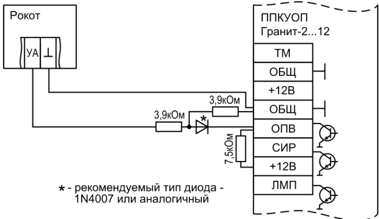
Рис.А2 Схема подключения «Рокот» к выходу «ОПВ» ППКУОП «Гранит-2,-3,-4,-5,-8,-12»
