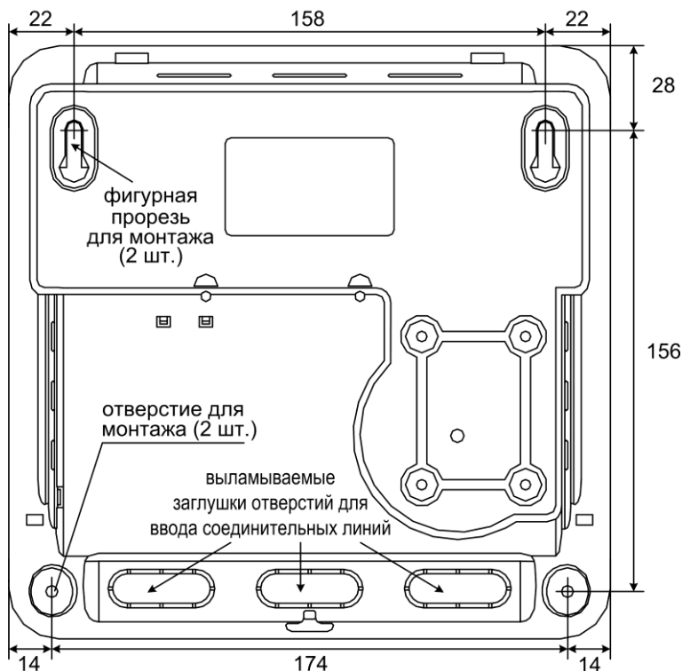
Рис.А7 Задняя стенка. Присоединительные размеры, расположение отверстий для крепежа
