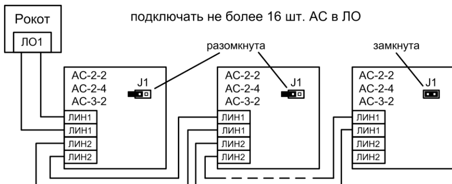
Рис.А5 Схема подключения акустических систем «АС-2-2», «АС-2-4», «АС-3-2» (параллельное соединение)
