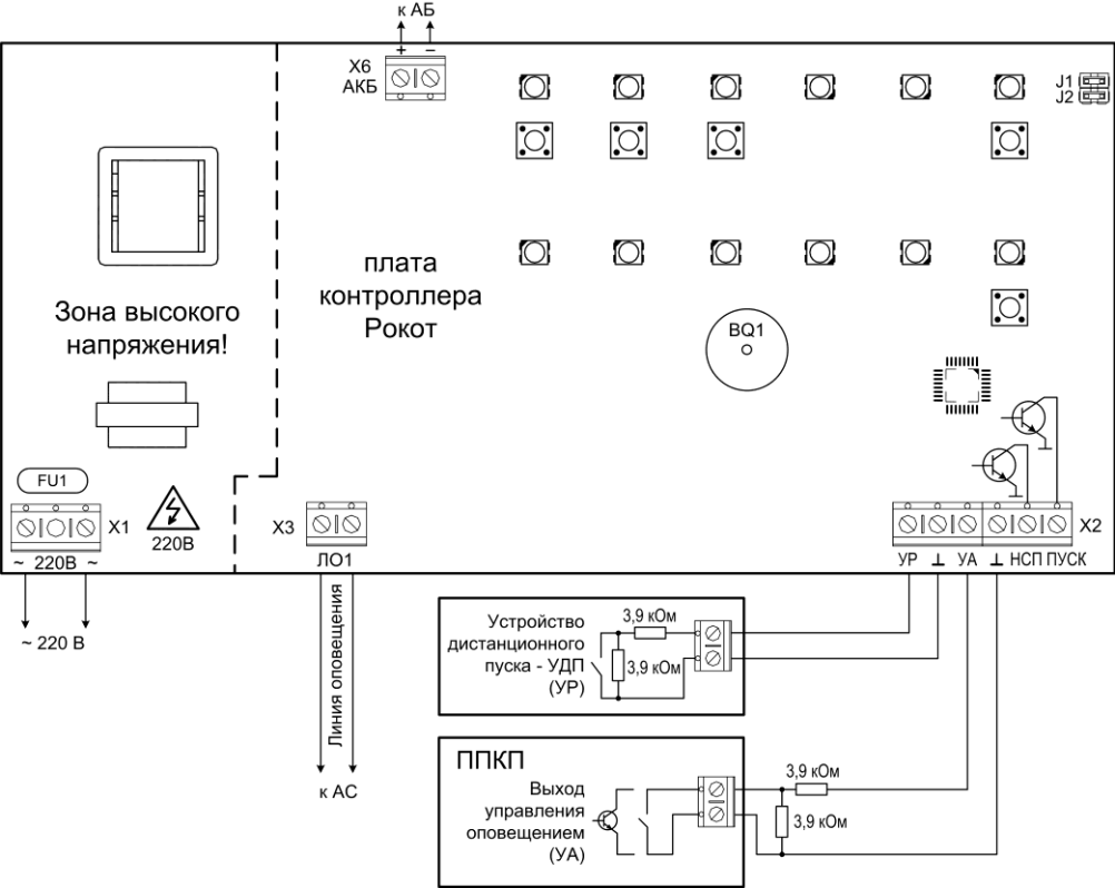
Рис.А1 Плата контроллера (вид со снятой панелью индикации и управления) и схема внешних подключений прибора «Рокот»
