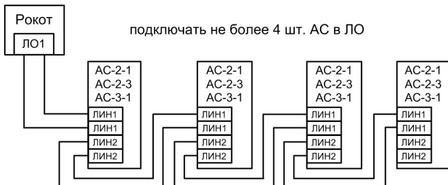
Рис.А3 Схема подключения акустических систем «АС-2-1», «АС-2-3», «АС-3-1» (параллельное соединение)
