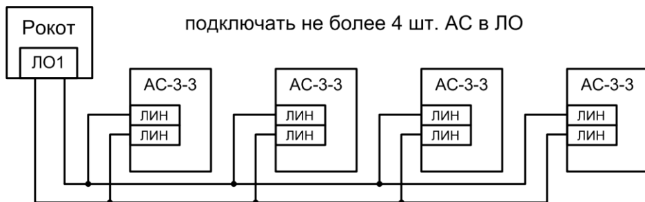
Рис.А4 Схема подключения акустических систем «АС-3-3» (параллельное соединение)
