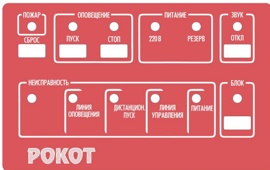
Рис.1 Панель индикации и управления прибора
