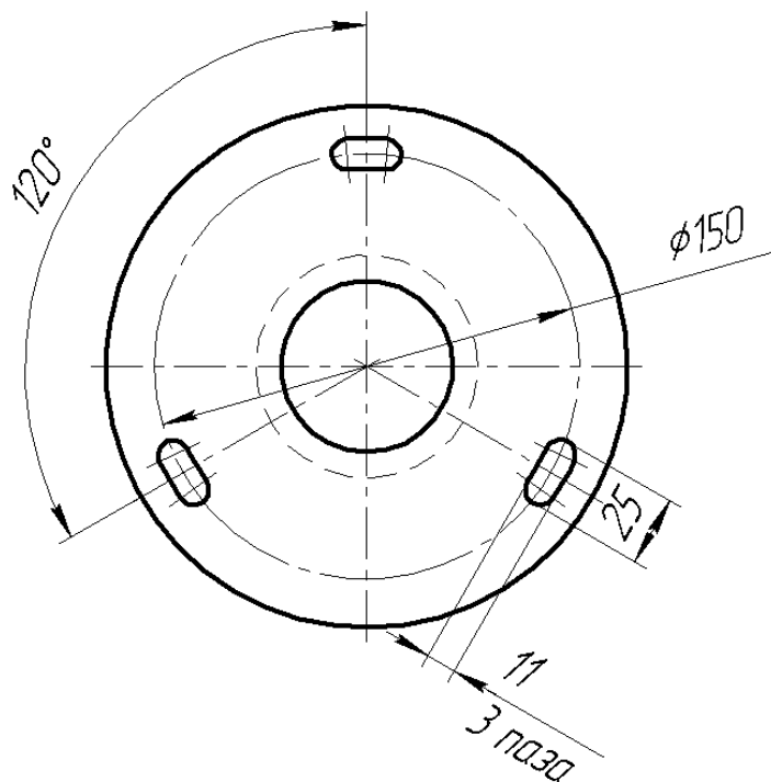
Установочные размеры калитки «Ростов - Дон К21»
