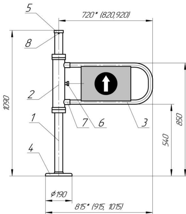
Габаритные и установочные размеры калитки «Ростов-Дон К21»
