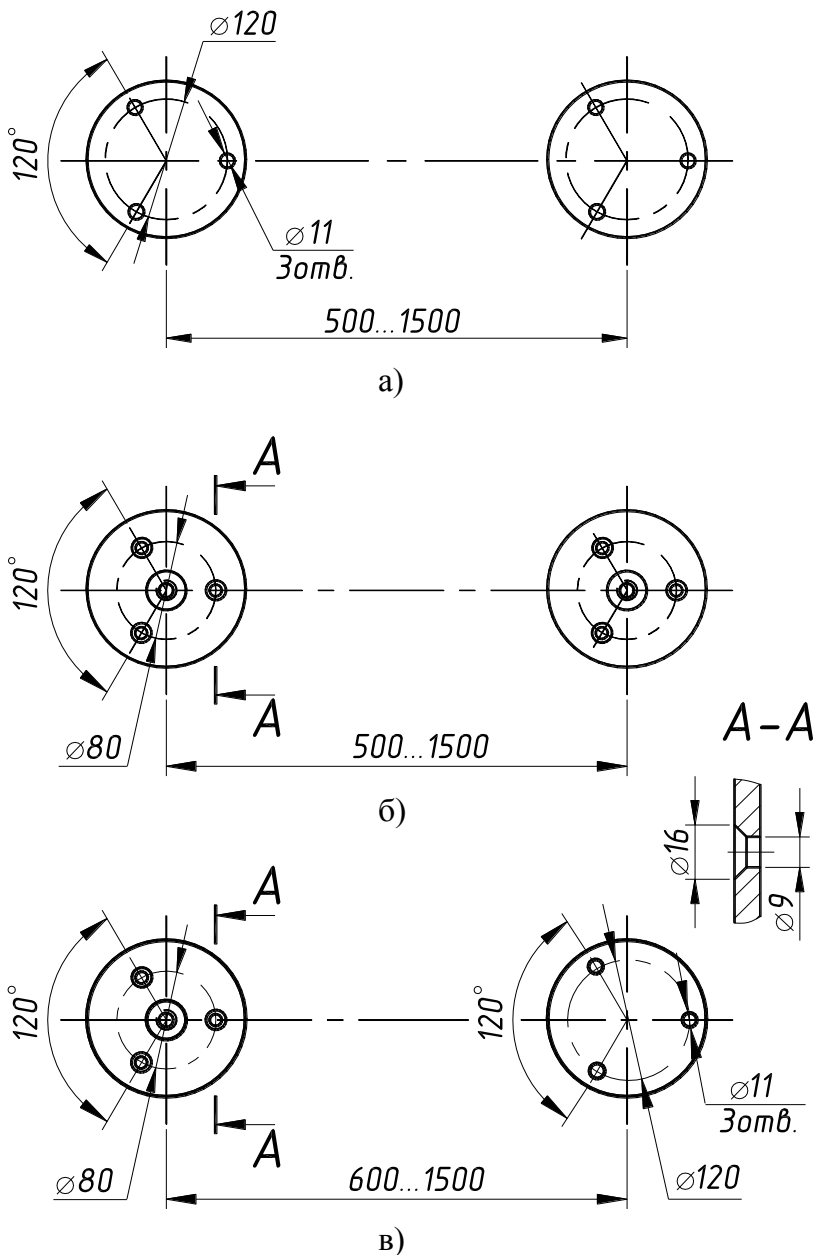
Рис. 18. Установочные размеры стоек стационарных ограждений:
