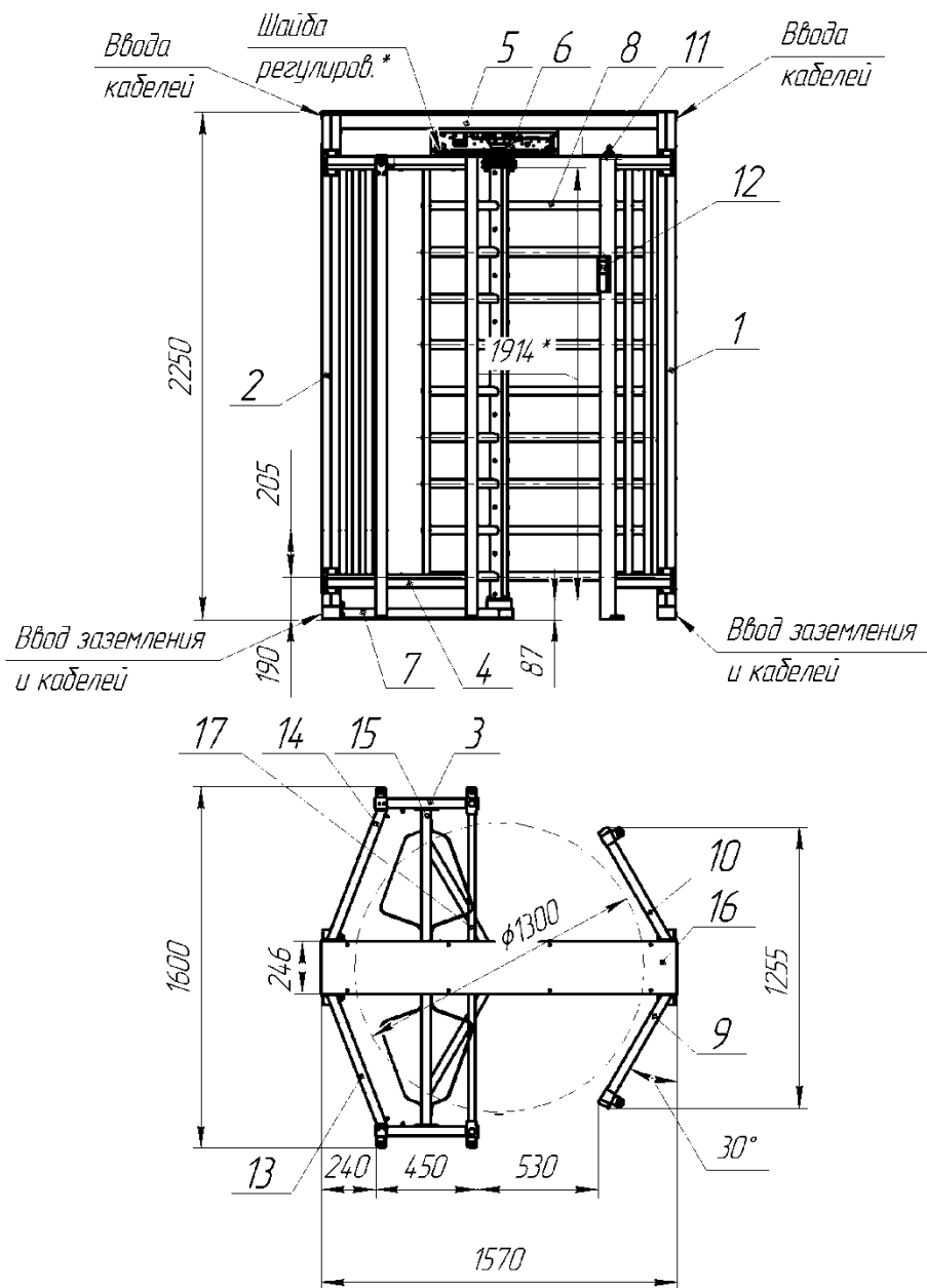
Габаритные размеры турникета «Ростов-Дон ПР1/ЗМ2»
