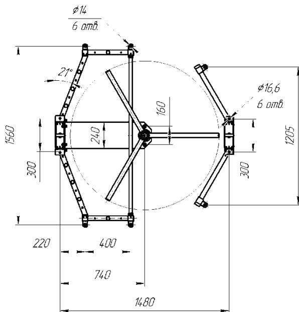
Установочные размеры турникета «Ростов-Дон ПР1/ЗМ2»
