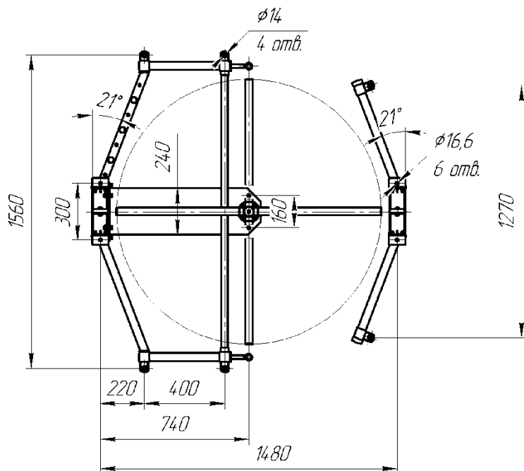
Установочные размеры турникета «Ростов-Дон ПР1/4М2»
