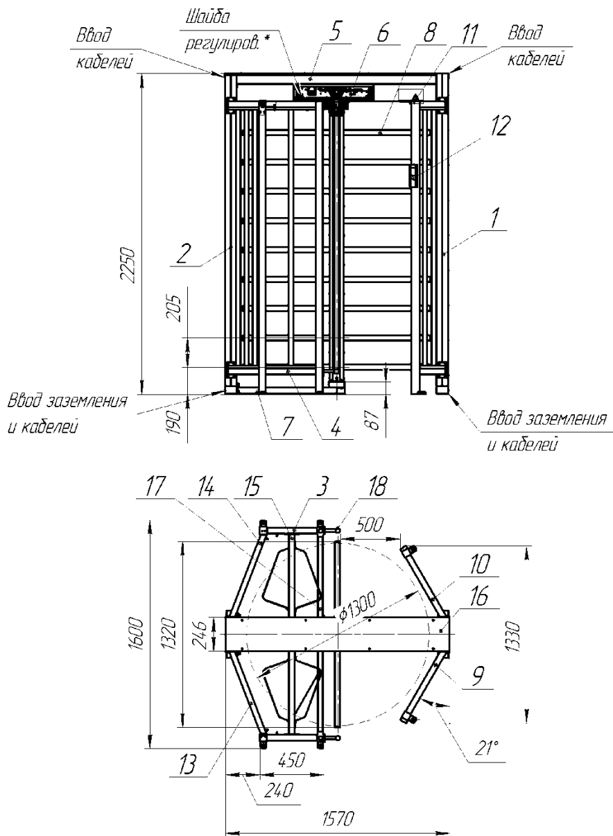
Габаритные размеры турникета «Ростов-Дон ПР1/4М2»
