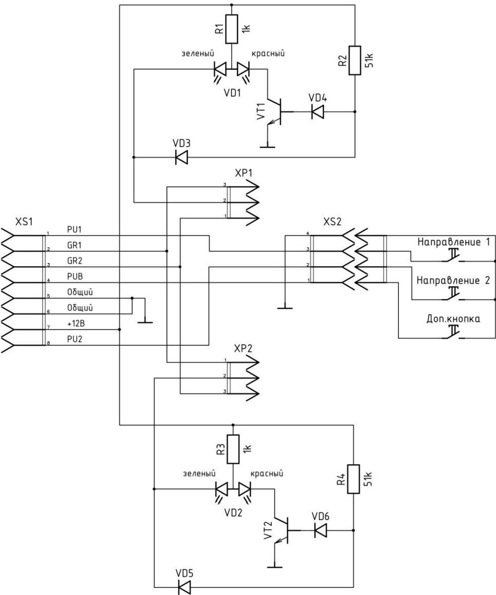
Схема электрическая принципиальная пульт дистанционного управления П2П-0-0Г
