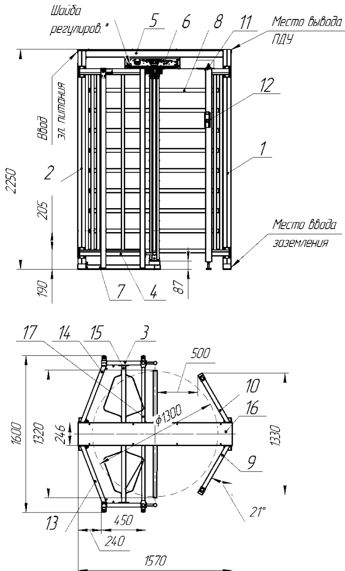
Габаритные размеры турникета «Ростов-Дон ПР1/4М2»
