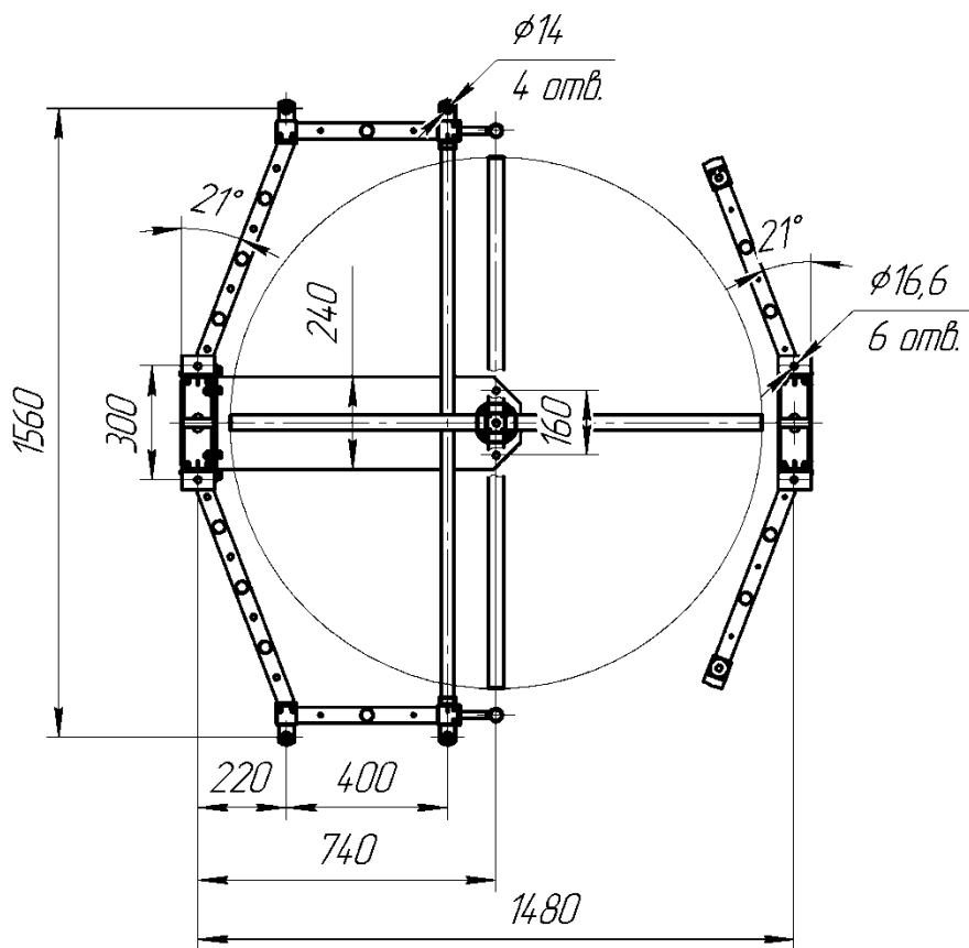
Установочные размеры турникета «Ростов-Дон ПР1/4М2»
