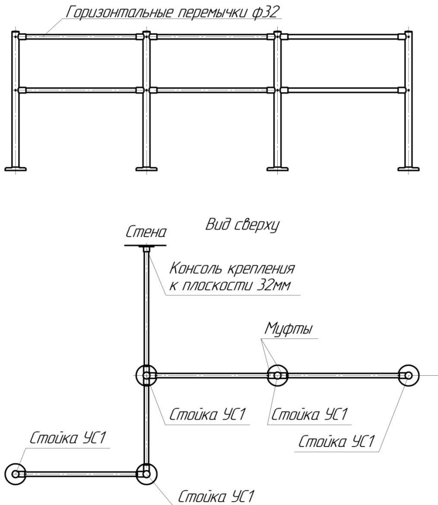
Пример компоновки ограждения ОС1-у
