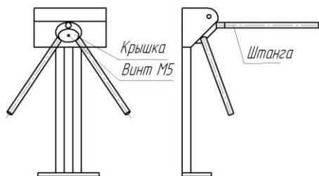
Рис.1 Установка штанг
