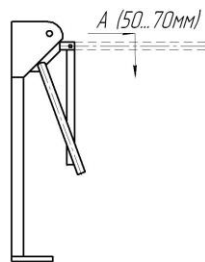
Рис.2 Штанга-антипаника
