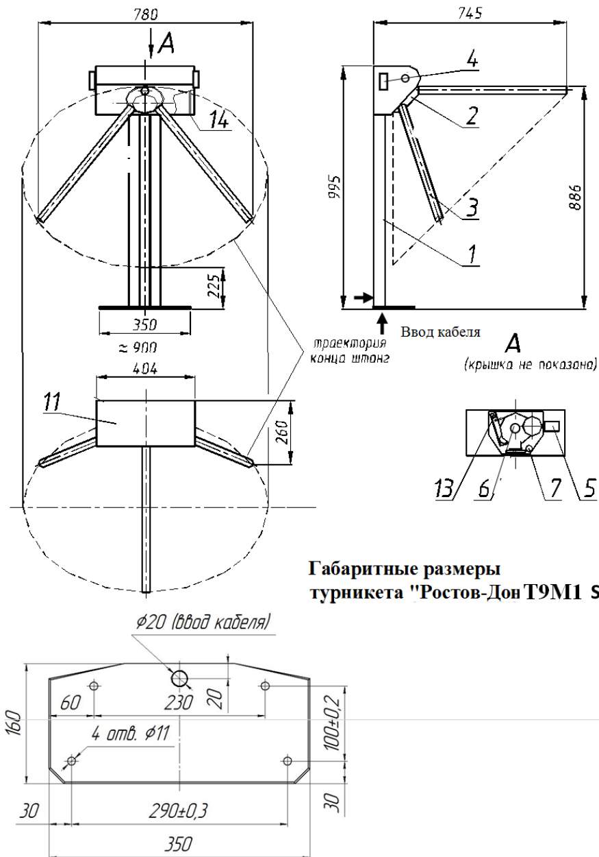
Установочные размеры турникета "Ростов-Дон Т9М1 Step"
