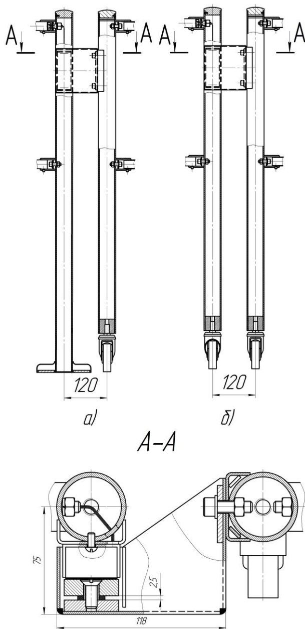
Рис. 12. Варианты электромагнитного замка: а) замок на стойке ограждения OC1; б) замок на стойке колесной OC2ак
