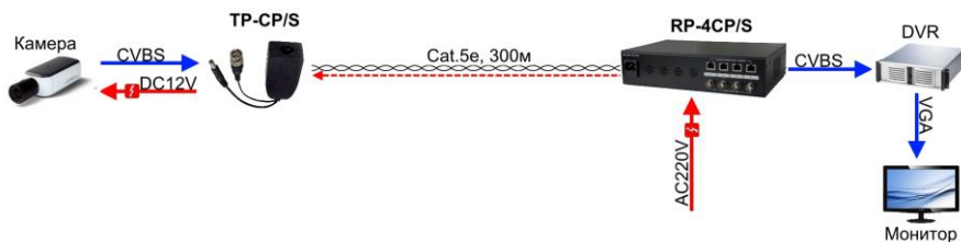
Рис. 4 Схема подключения TP-CP/S к RP-4CP/S, RP-8CP/S, RP-16CP/S
