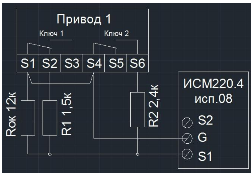
Схема подключения концевиков контроля положения привода к безадресному шлейфу ИСМ220.4 исп.08
