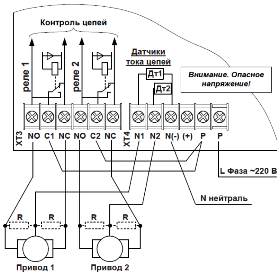
Схема подключения двух реверсивных приводов постоянного тока типа "Белимо"
