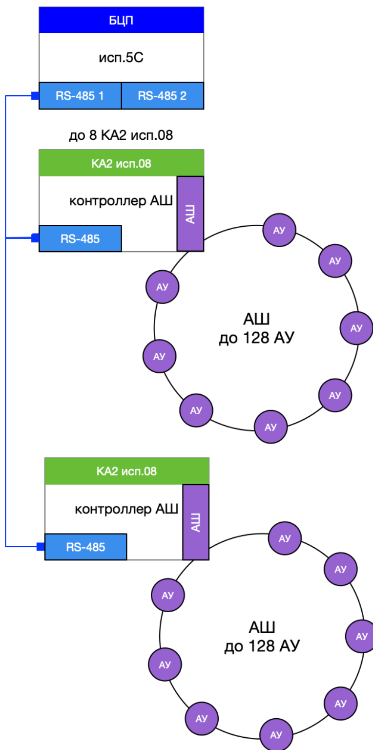
Рис. 1 Подключение двух кольцевых АШ в системе ИСБ ИНДИГИРКА
