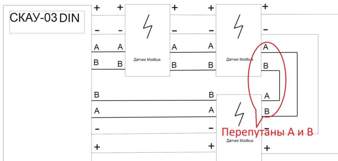
Рис.7 Неправильное подключение Modbus RTU интерфейса
