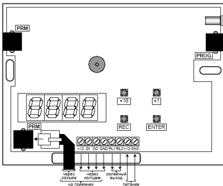
Рис. 4. Монтажная схема пульта при внутреннем подключении
