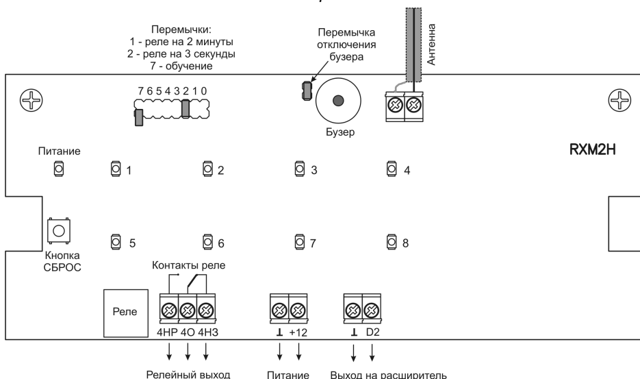
Рис. 2. Монтажная схема приемника
