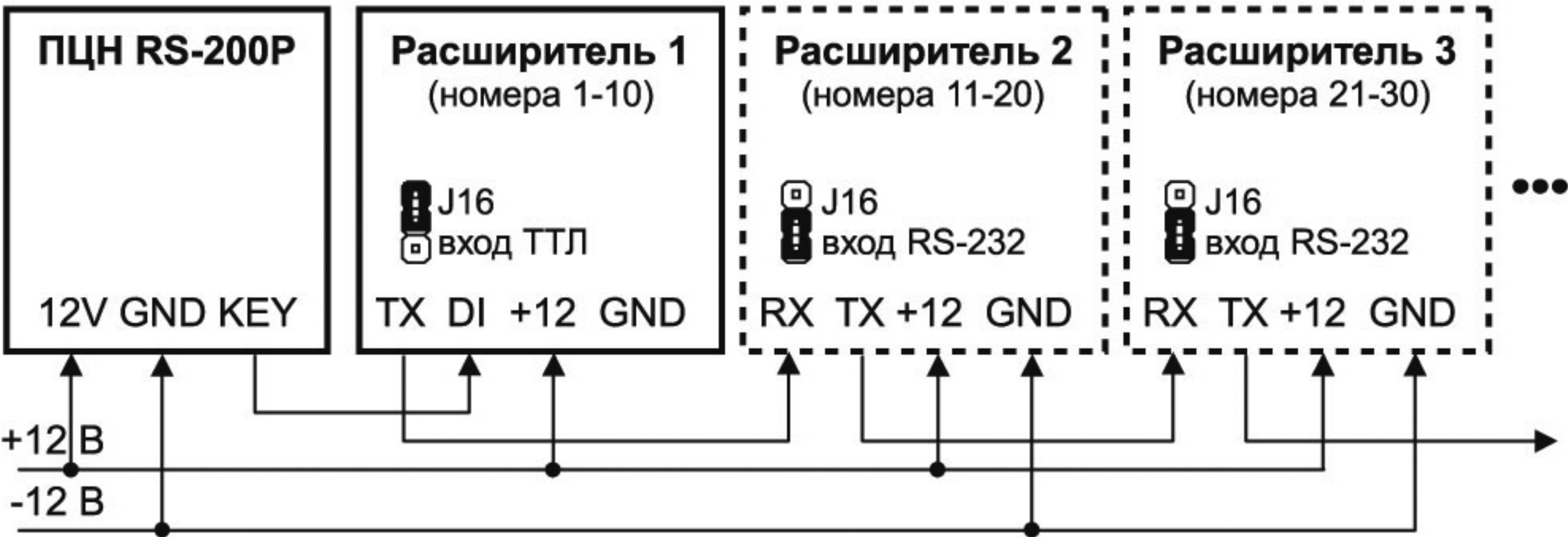
Подключение расширителя к ПЦН RS-200P (до 16 шт.)
