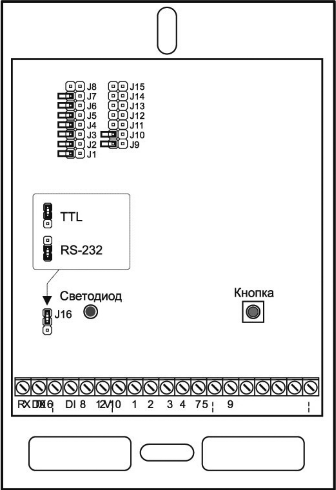
Монтажная схема расширителя
