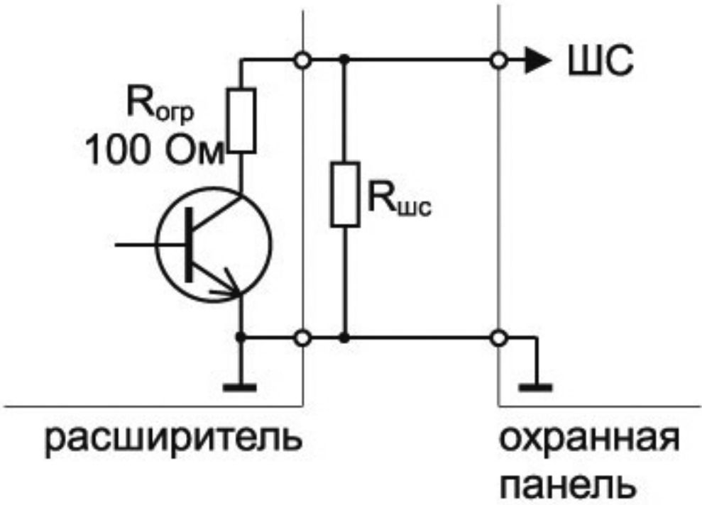
Пример монтажа шлейфа сигнализации
