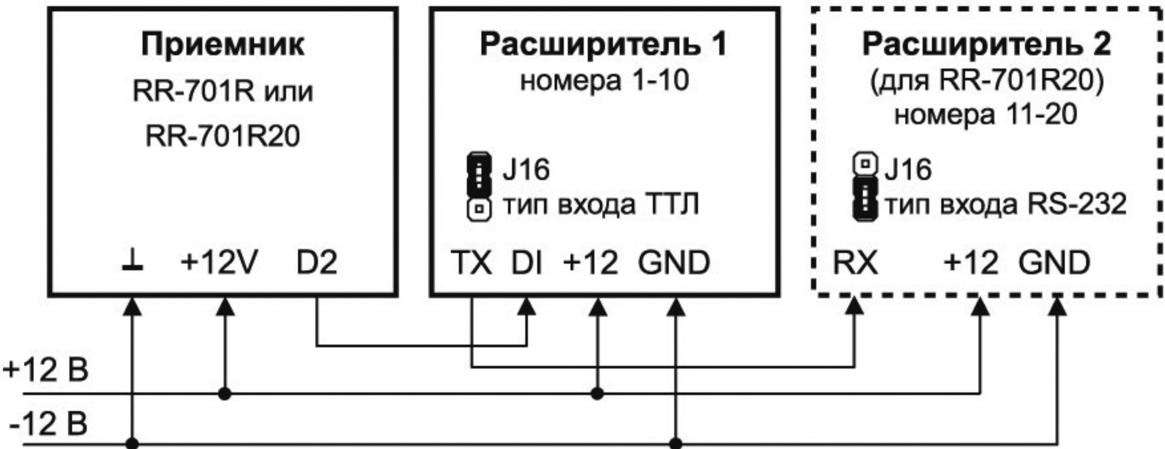
Подключение расширителя к приемникам RR-701
