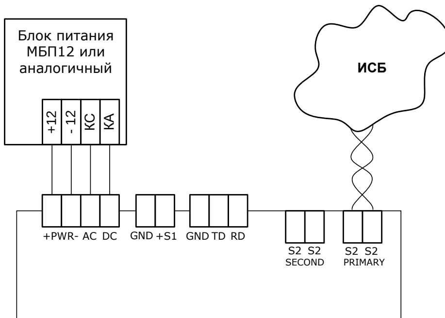
Рисунок 1 Подключение РРОП-И
