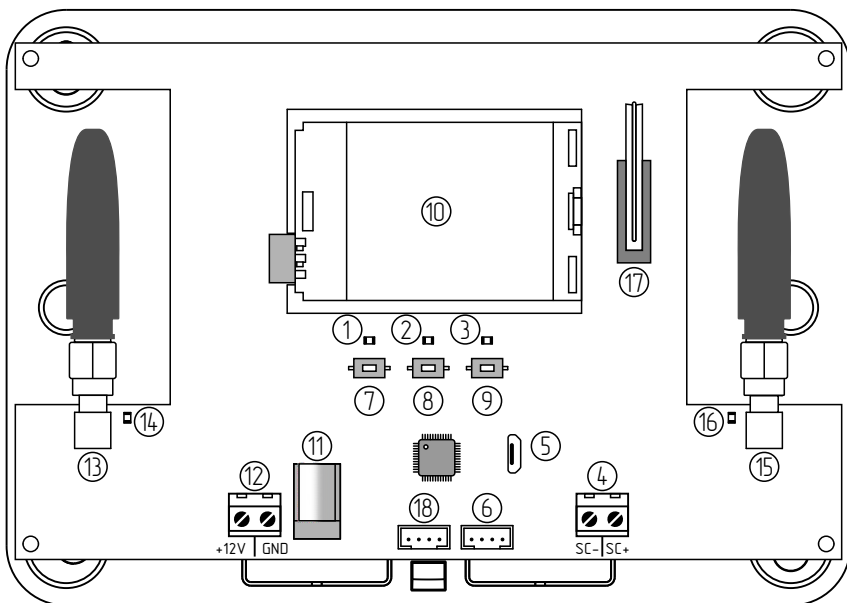
Рисунок 1. Плата ретранслятора
