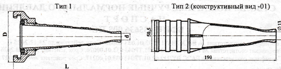
Рисунок 1. Стволы РС
