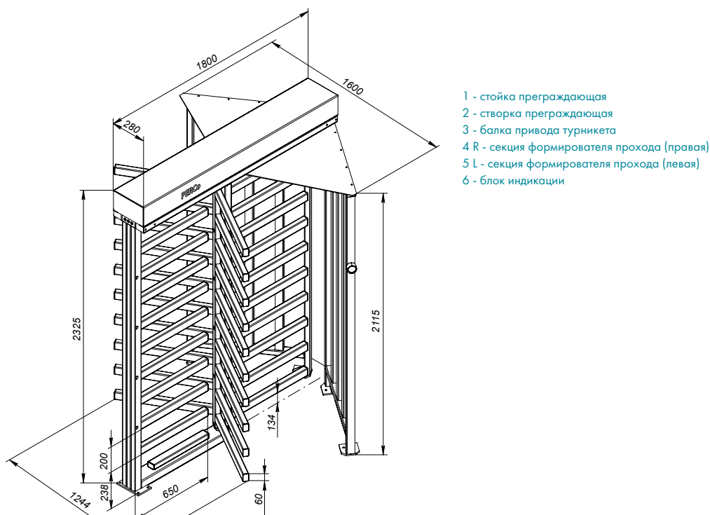
Габаритные размеры турникета без крыши
