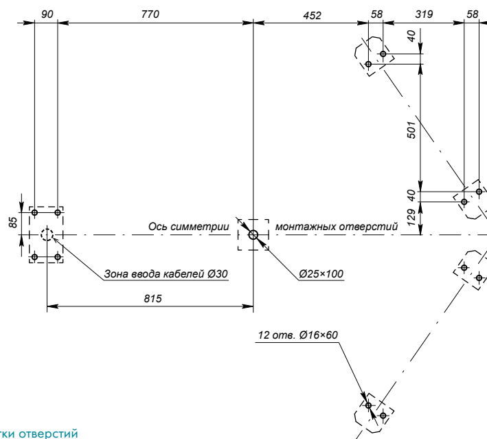
Схема разметки отверстий
