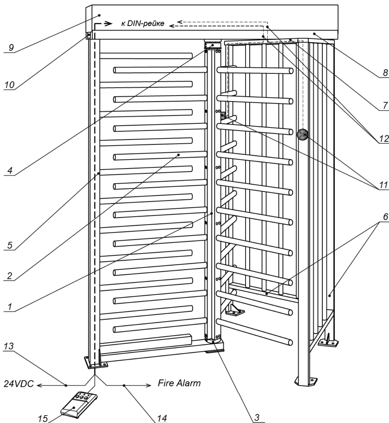
Рисунок 2. Устройство турникета:
