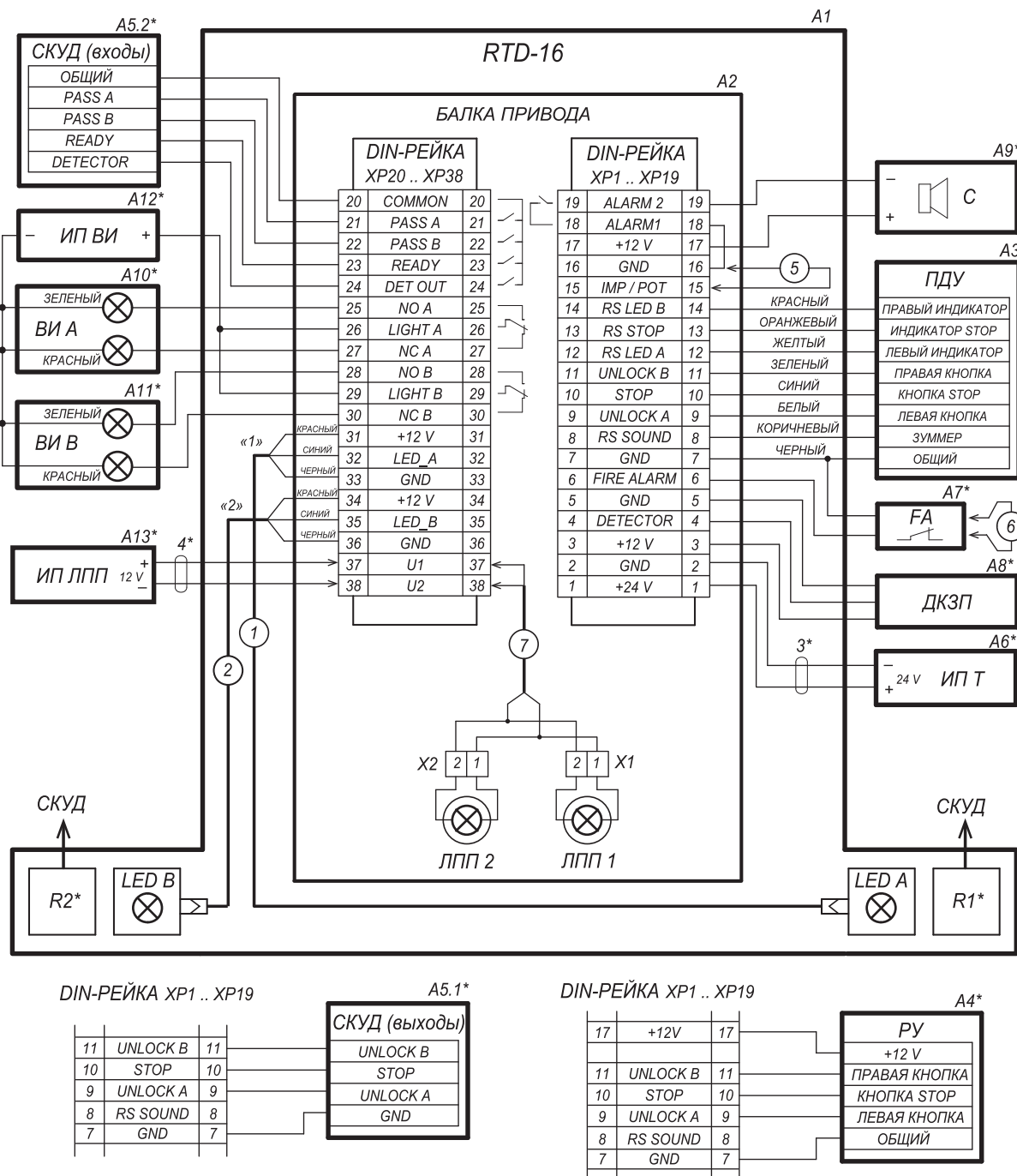
Схема внешних подключений к турникету RTD-15
