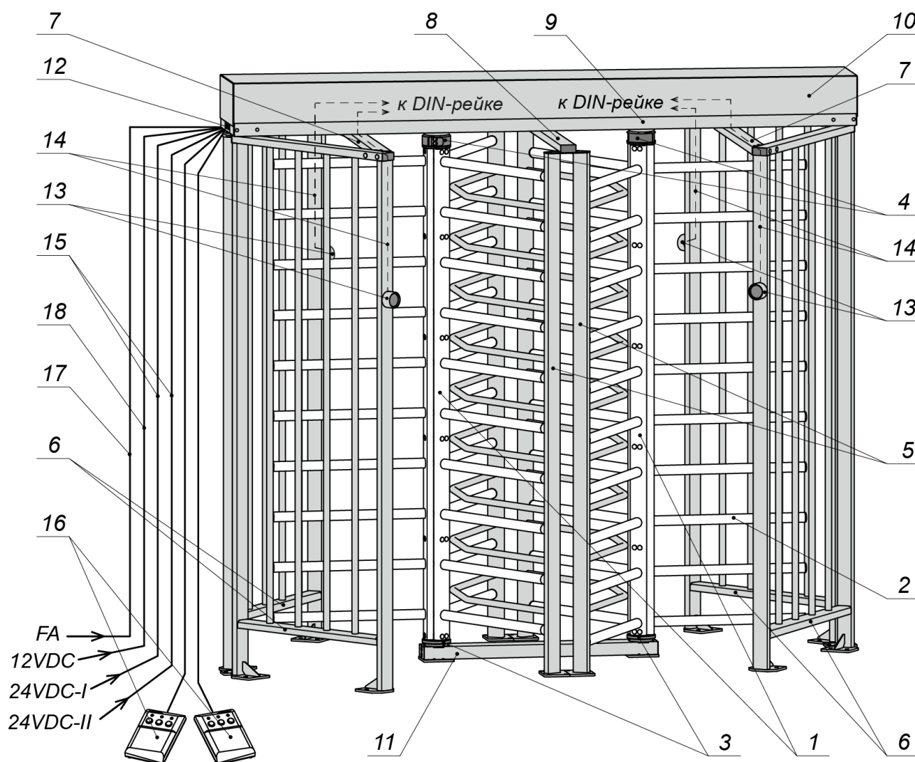
Рисунок 2. Устройство турникета:
