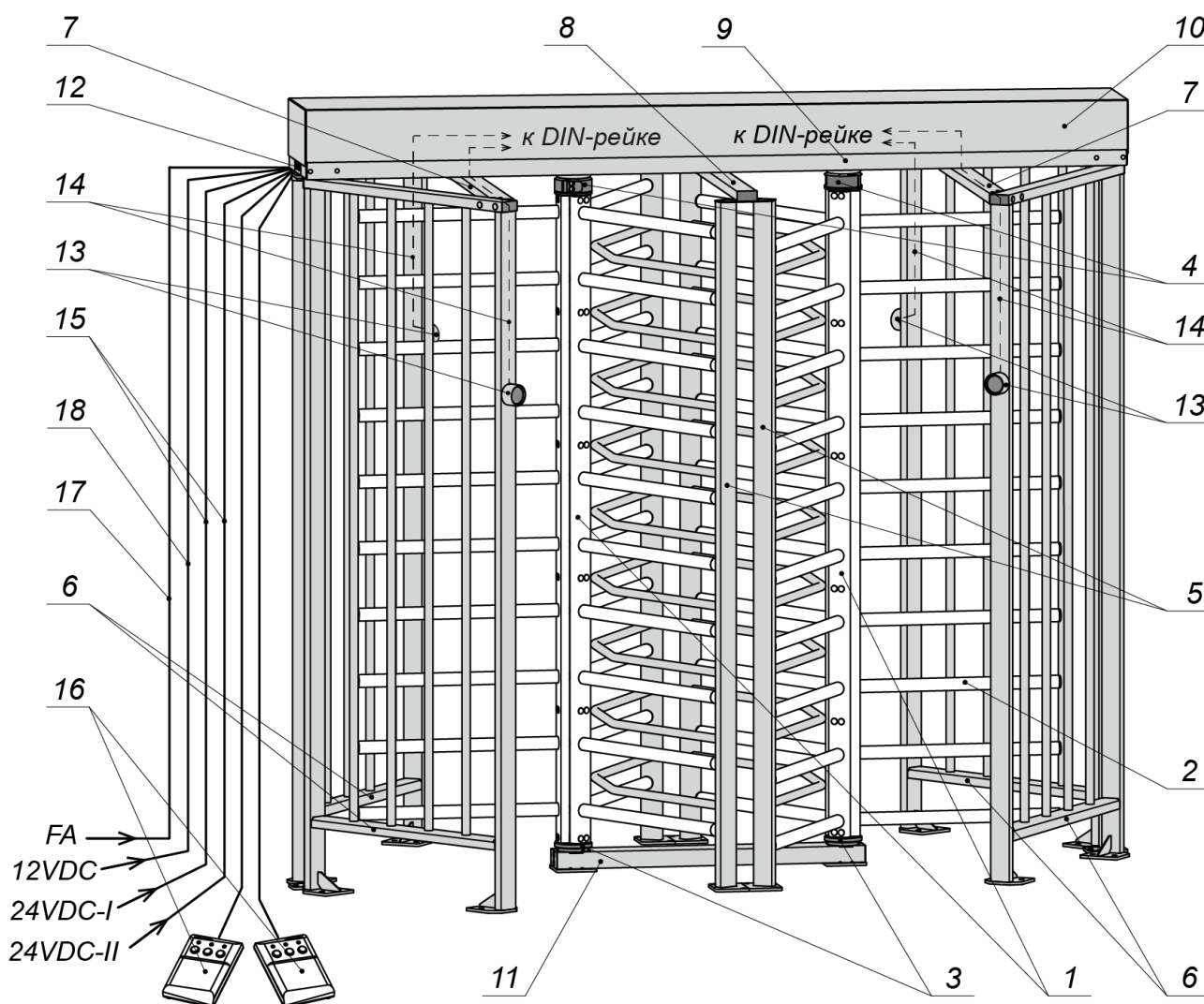
Рисунок 2. Устройство турникета:
