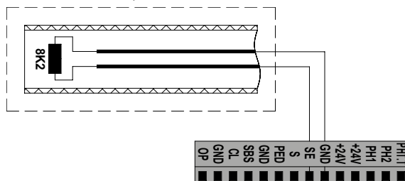
Рисунок 17. Схема подключения резистивной кромки безопасности 8,2 кОм
