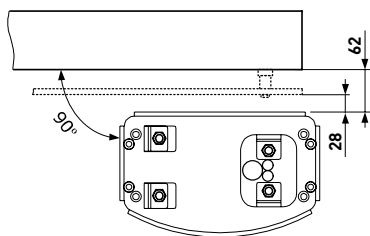
Рисунок 4. Расположение монтажного основания относительно створки
