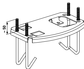
Рисунок 3. Монтажное основание
