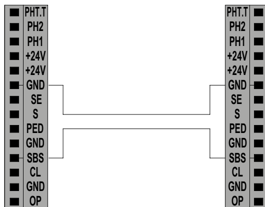
Рисунок 19. Схема подключения двух электронных блоков управления для синхронизации работы двух приводов
