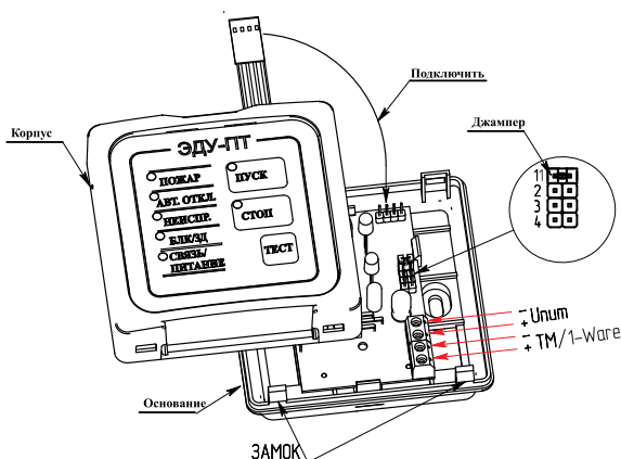
Рисунок 9. Установка ЭДУ-ПТ.
