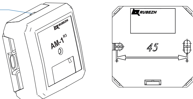
Рисунок 10. Установка АУ в корпусе типа AM-1.
