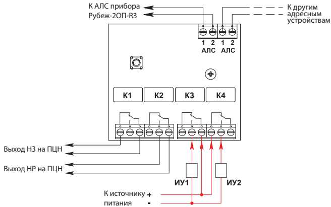
Рисунок 16. Внешние подключения к релейному модулю РМ-4 прот.Р3
