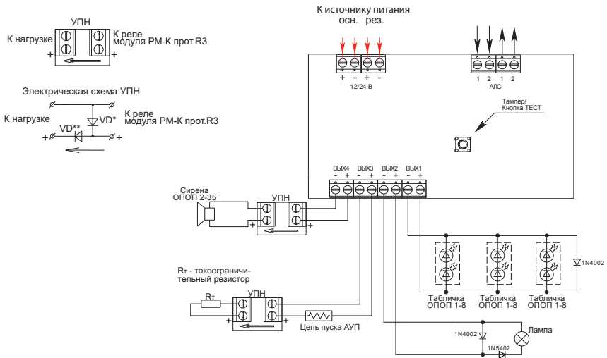
Рисунок 17. Внешние подключения к релейному модулю РМ-4К прот.Р3
