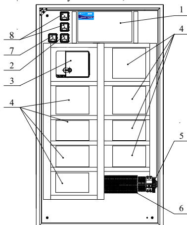
б) Рубеж-МК2
