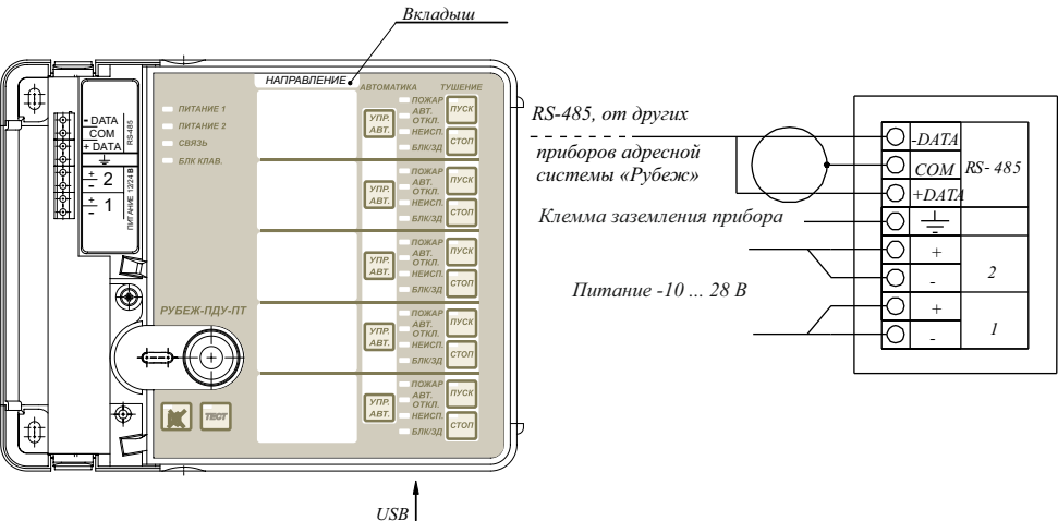
Рисунок 1 – Внешний вид и схема подключения прибора
