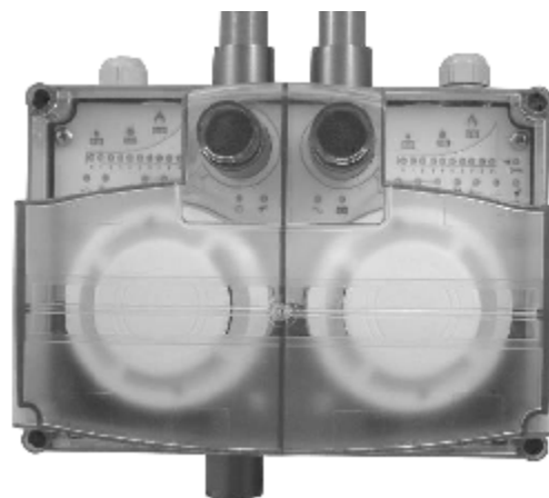
Рис. 25. Центральный блок аспирационного извещателя LASD-2
