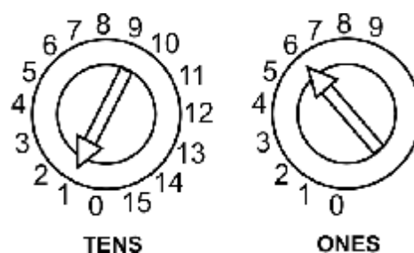
Рис. 6. Декадные переключатели для установки адресов
