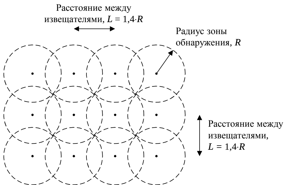
Рис. 48. Схема размещения дымовых или тепловых извещателей в помещении по "квадратной решетке"
