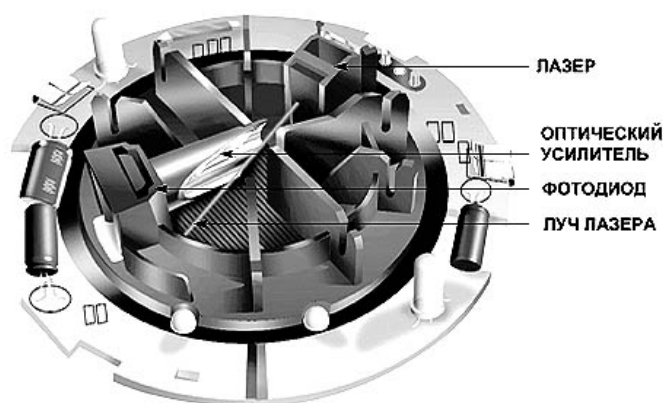
Рис. 16. Дымовая камера лазерного извещателя 7251
