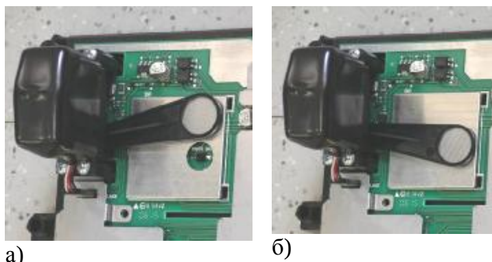
Рис. 22. Положение оптического фильтра а) в рабочем режиме, б) при тестировании
