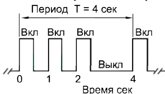
Рис. 46. Временная диаграмма стандартного сигнала пожарной тревоги
