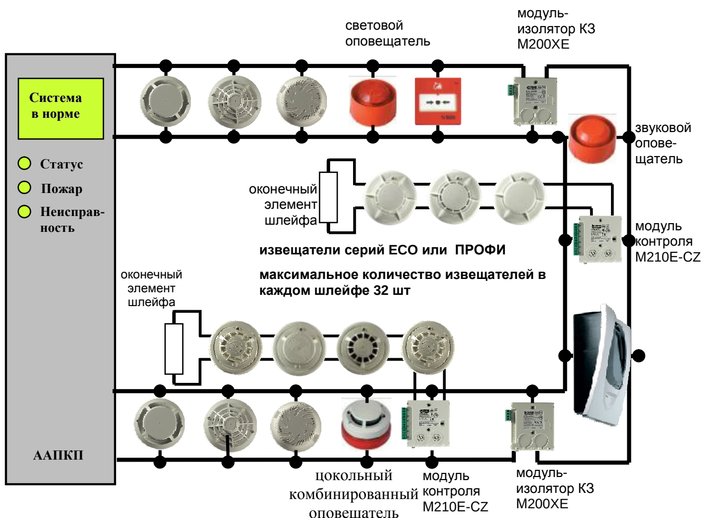
Рис. 5. Упрощенная структура кольцевого шлейфа адресно-аналоговой системы
