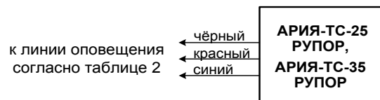
Рис. Схема подключения
