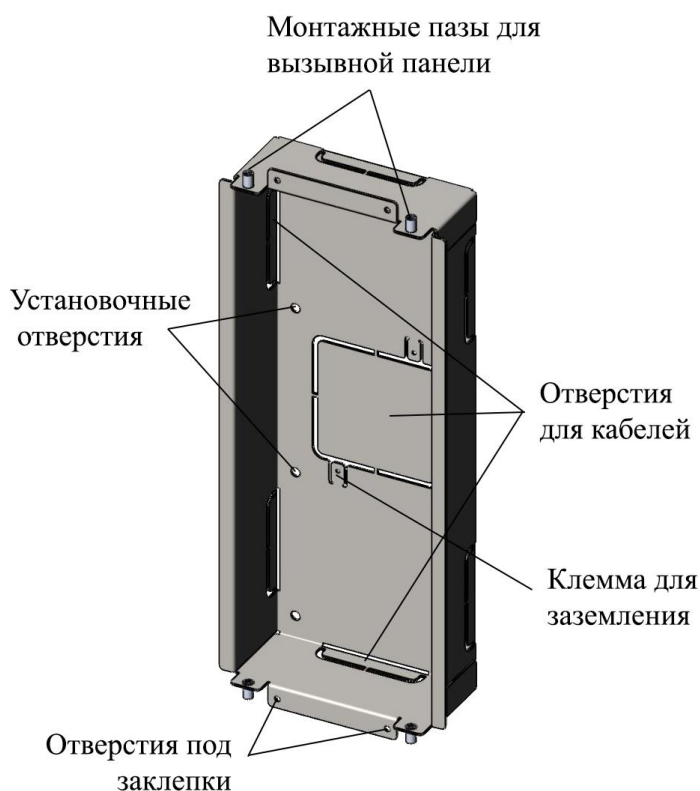
Рисунок 1 – Крепление врезное
