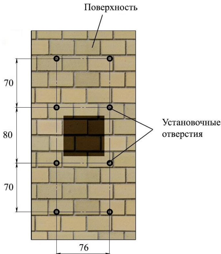
Рисунок 4 — Разметка установочных отверстий
