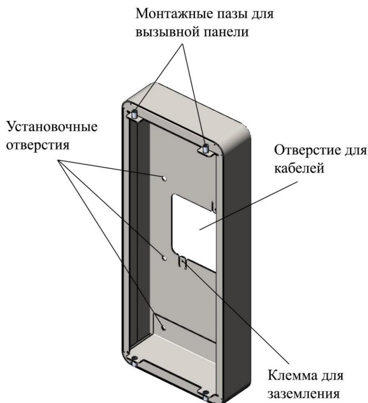
Рисунок 1 – Крепление накладное
