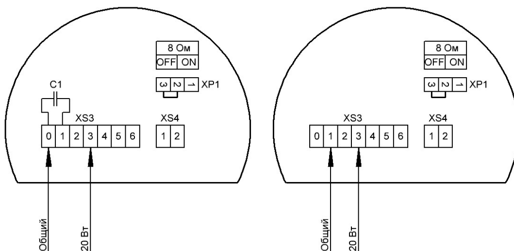
Рисунок Б2 – Схема подключения ГВП-Exd-20
