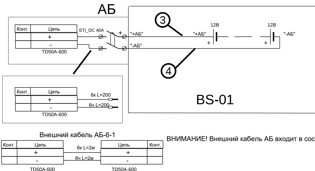
Рисунок 3 – Схема соединений для BS-01
