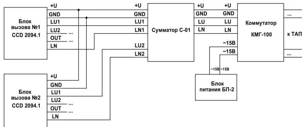
Рис. 2а Схема подключения сумматора, при величине сопротивления проводов, соединяющих блок вызова с сумматором не более 6 Ом для CCD 2094.1 и не более 1,5 Ом для CCD 2094.1/РК
