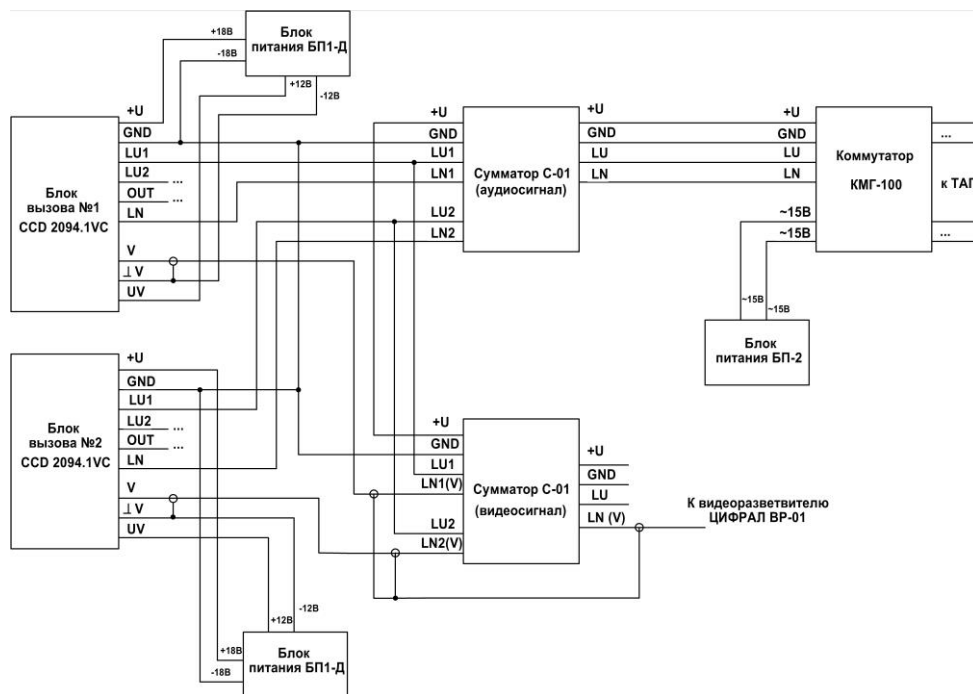
Рис. 3б Схема подключения сумматоров, для блоков вызова с видеосигналом при величине сопротивления проводов, соединяющих блок вызова с сумматором более 6 Ом для CCD 2094.1/VC и более 1,5 Ом для CCD 2094.1/PKVC (длинная линия)
