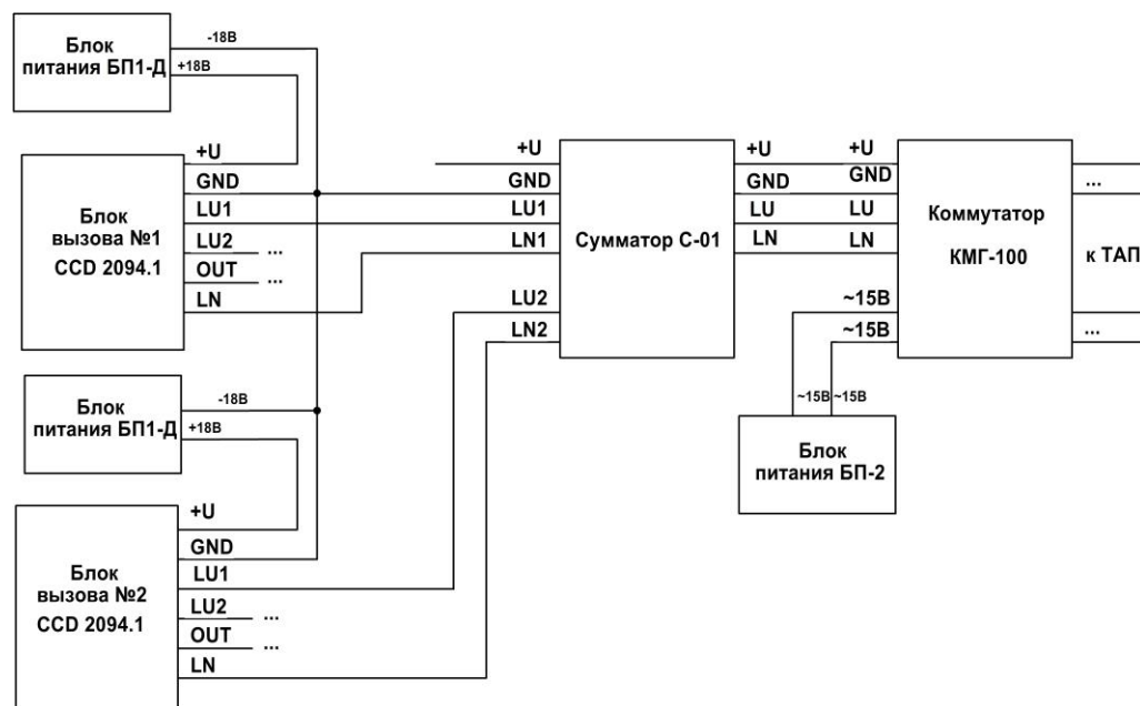
Рис. 2б Схема подключения сумматора с дополнительным источником питания, при величине сопротивления проводов, соединяющих блок вызова с сумматором более 6 Ом для CCD 2094.1 и не более 1,5 Ом для CCD 2094.1/РК (длинная линия)
