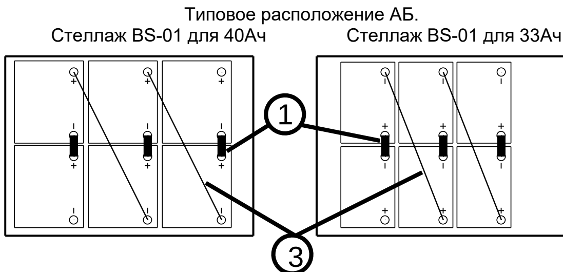
Рисунок 2 – Типовое расположение аккумуляторных батарей в стеллаже BS-01
