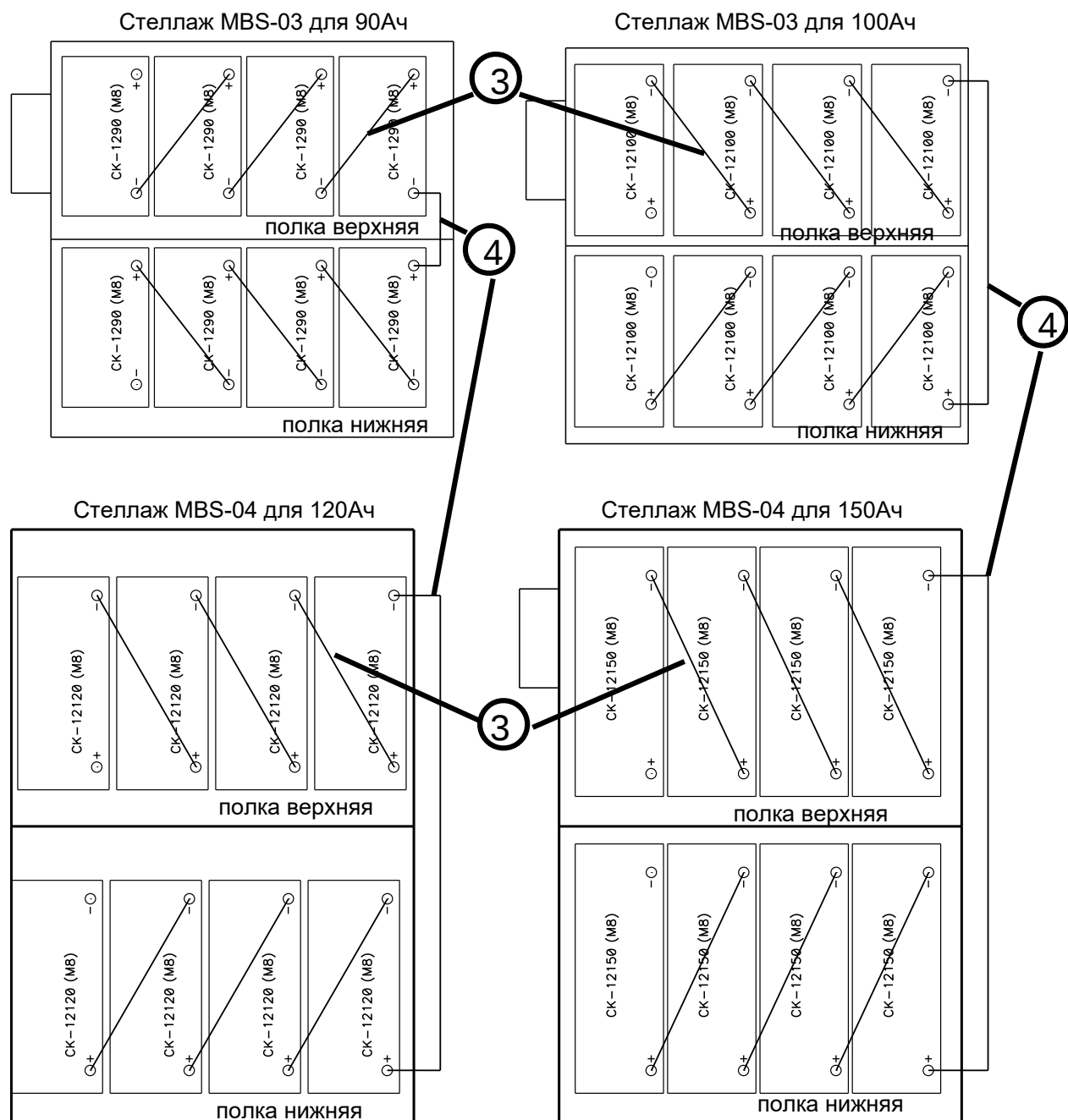
Рисунок 2 – Типовое расположение АБ
