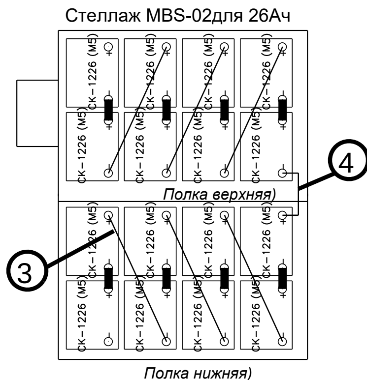
Рисунок 2 – Типовое расположение АБ
