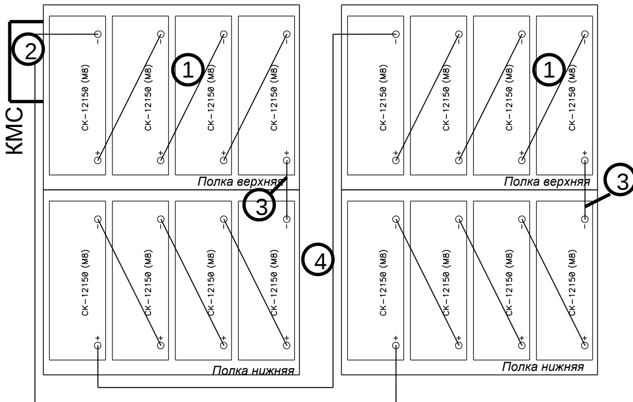
Рисунок 3 – Батарейный комплект S-20-4 для стеллажа MBS-04
