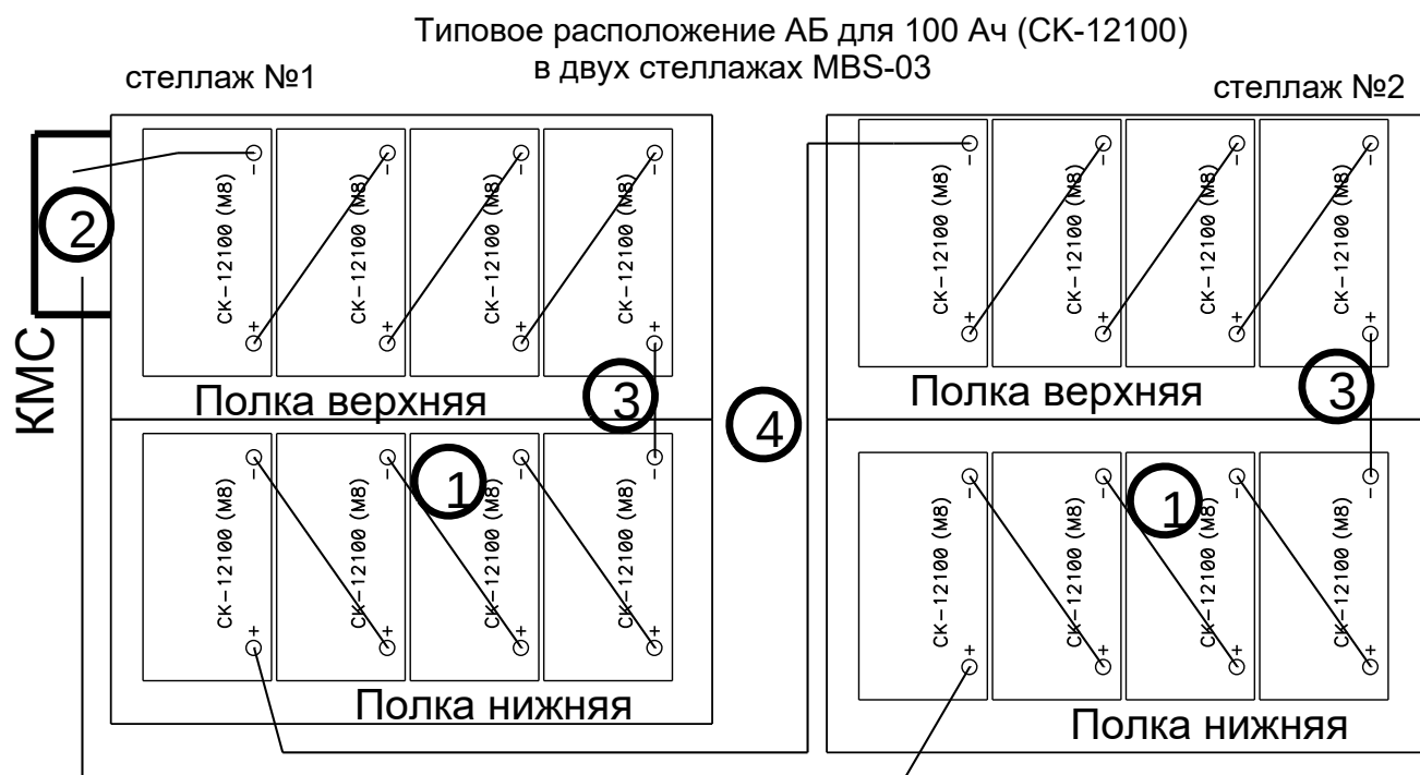
Рисунок 2 – Батарейный комплект S-20-4 для стеллажа MBS-03
