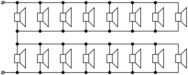
Подключение шестнадцати акустических оповещателей Z а =8 Ом, P н =3Вт; P вых ≈1,5Вт/оповещатель – рис.4
