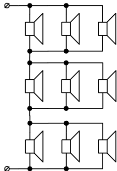
Подключение девяти акустических оповещателей Z_{ли}=4\text{ Ом} , P_{ли}=3\text{ Вт} ; P_{выс}\approx 1,65\text{ Вт/оповещатель} – рис. 7
