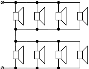
Подключение восьми акустических оповещателей Z а =4 Ом, P н =3Вт; P вых ≈3Вт/оповещатель – рис.3
