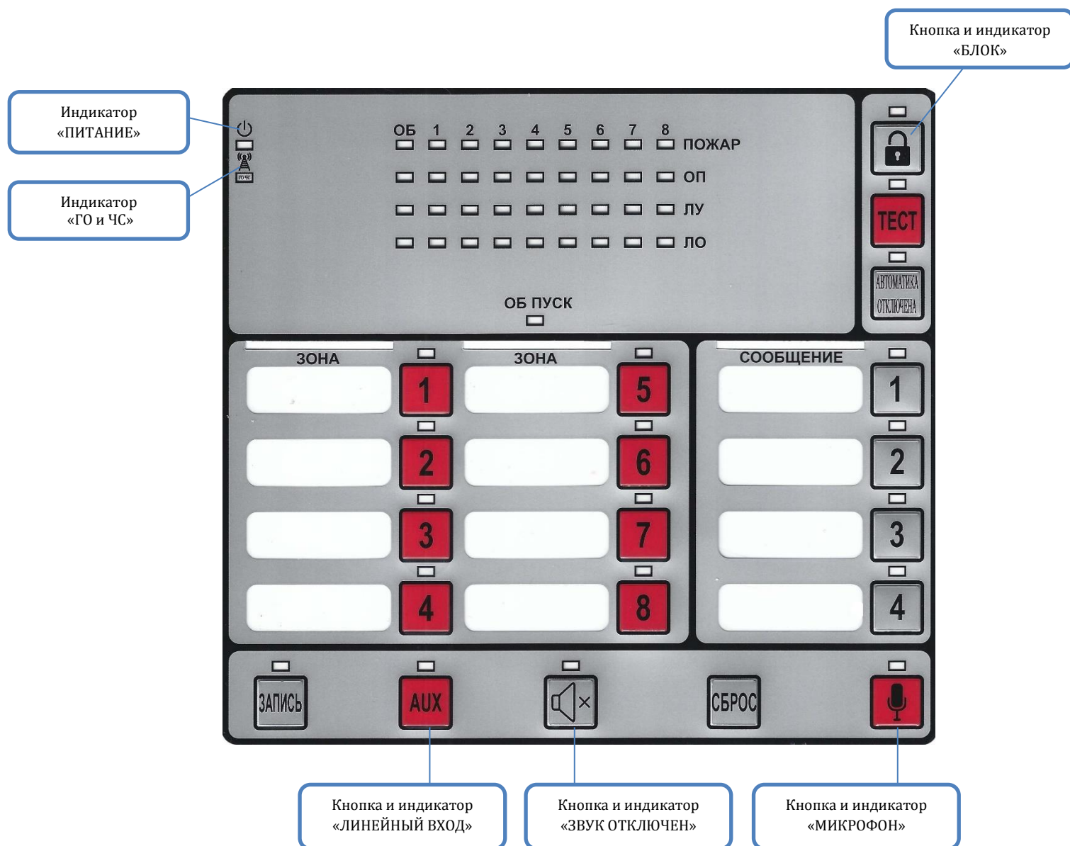
Рисунок 1. Органы управления и индикации блока управления
