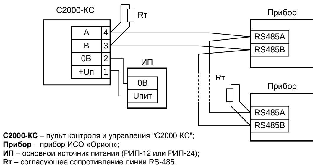
Рисунок 5 Типовая схема подключения пульта "С2000-КС" при эксплуатации
