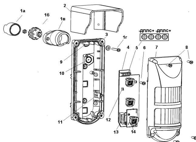
Рисунок 1 – Конструкция извещателя
