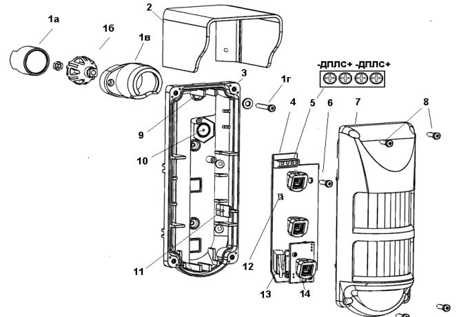
Рисунок 1 – Конструкция извещателя
